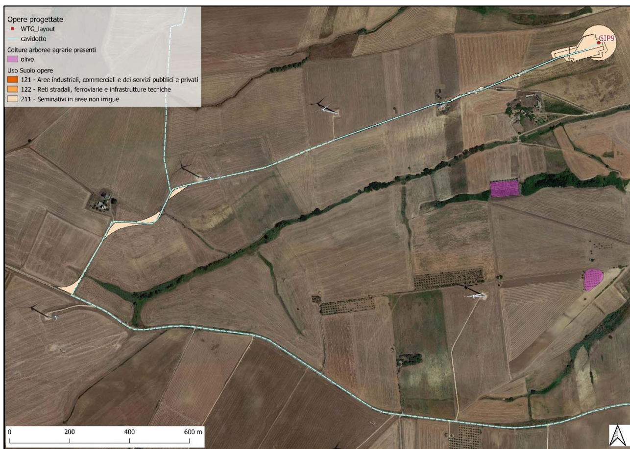
Figura 21 - Particolare della classificazione di suo del suolo, come da CTR, per l'aerogeneratore 9
