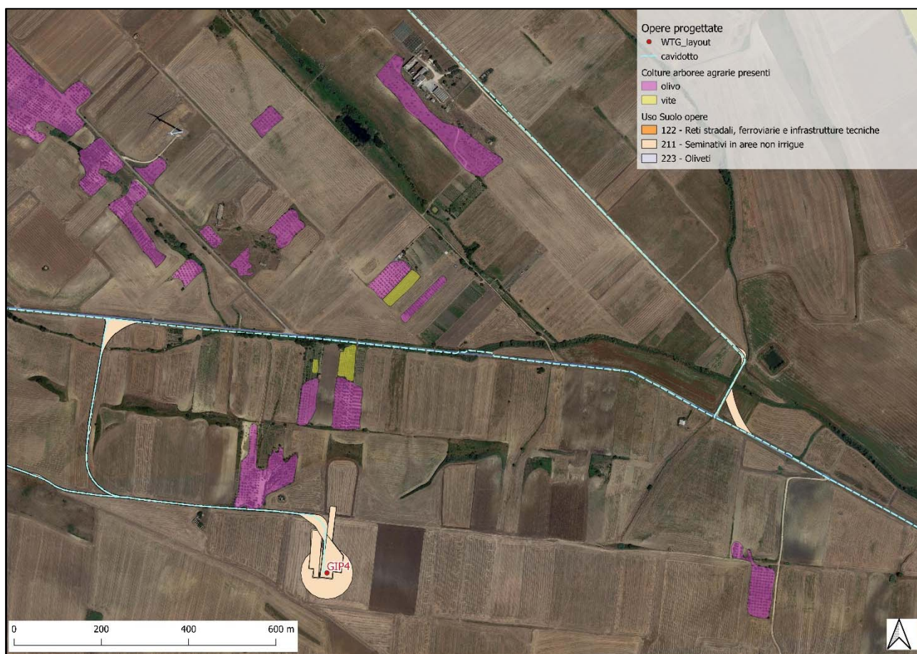
Figura 13 – Particolare della classificazione di suo del suolo, come da CTR, per l’aerogeneratore 4
