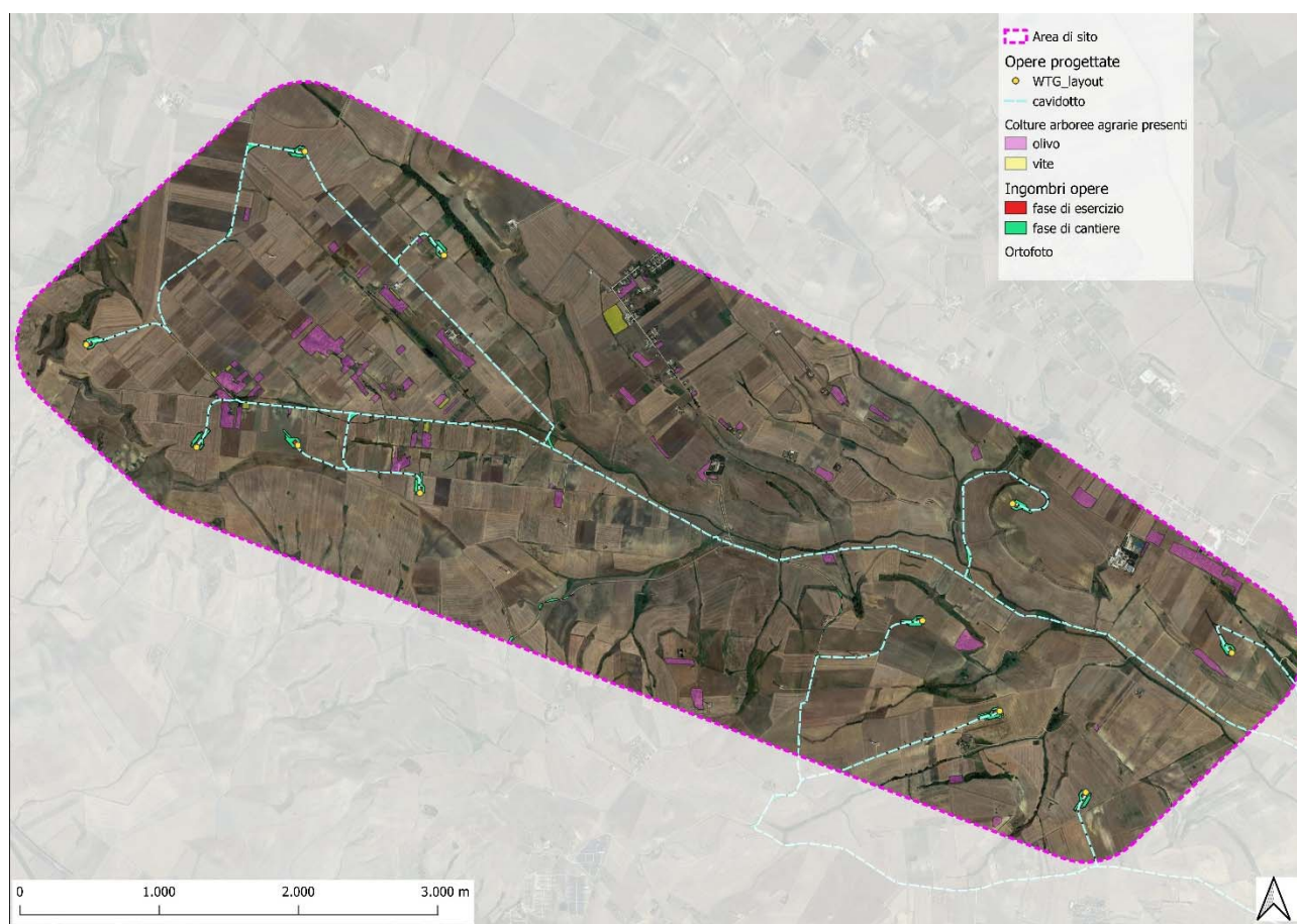
Figura 9 – Localizzazione degli ingombri presenti rispetto le colture arboree agrarie rinvenibili nell'area di sito
