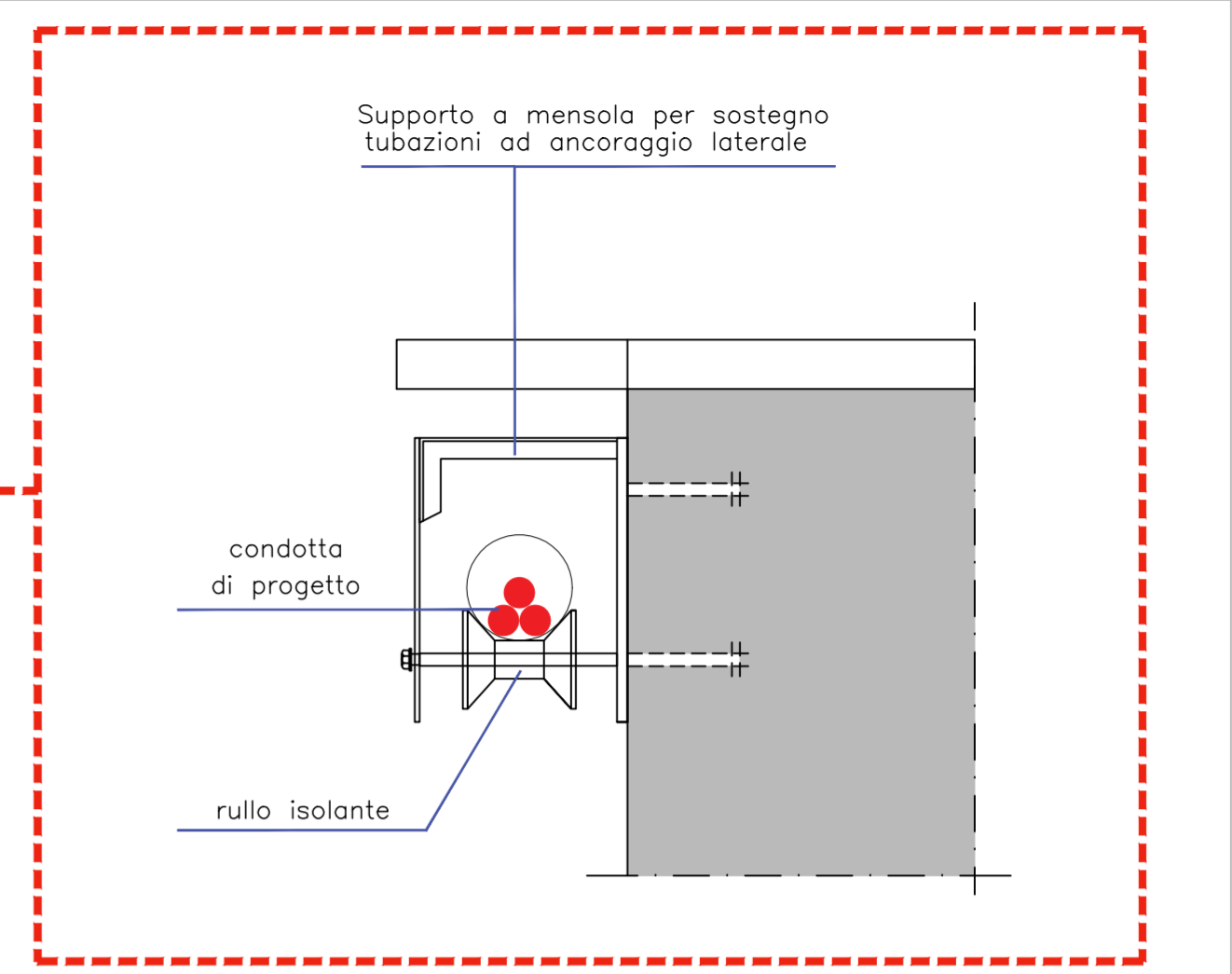
Dettaglio supporto (scala 1:50)
