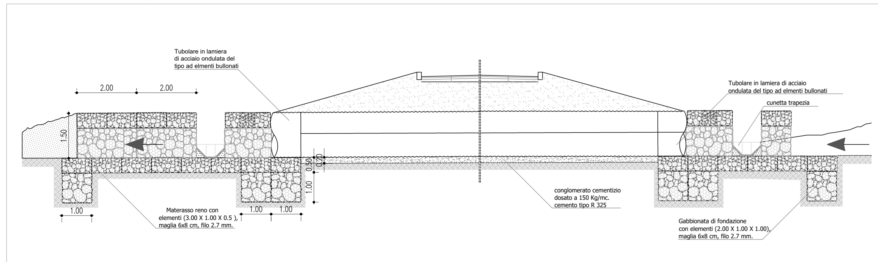
SEZIONE TIPOLOGICA TOMBINO IDRAULICO DI PROGETTO Sezione trasversale (scala 1:100)
