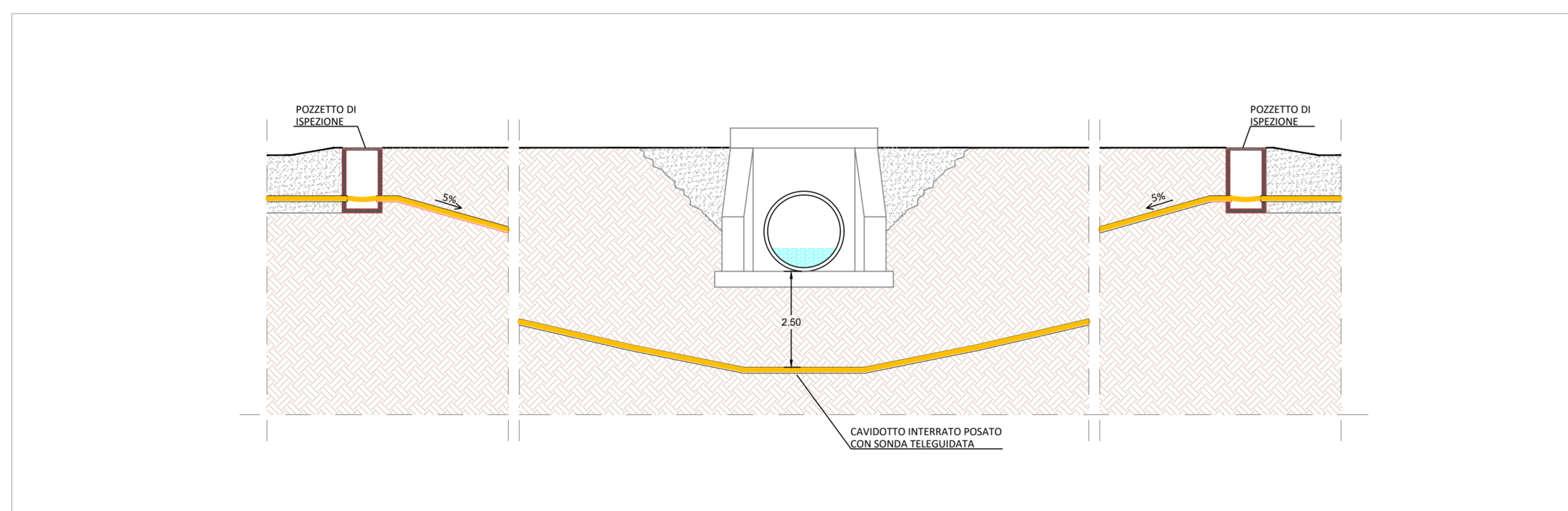
SEZIONE TIPOLOGICA DI RISOLUZIONE DELL'INTERFERENZA TRA CAVO MT E PONTICELLI MEDIANTE T.O.C. Sezione trasversale (scala 1:100)
