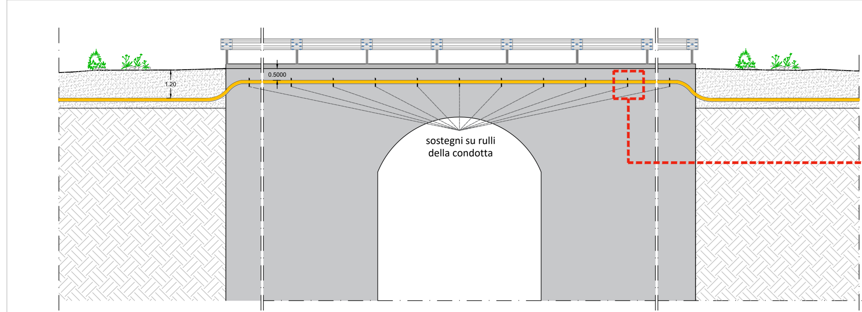
SEZIONE TIPOLOGICA DI RISOLUZIONE DELL'INTERFERENZA TRA CAVO MT E VIADOTTO MEDIANTE STAFFAGGIO Sezione trasversale (scala 1:100)
