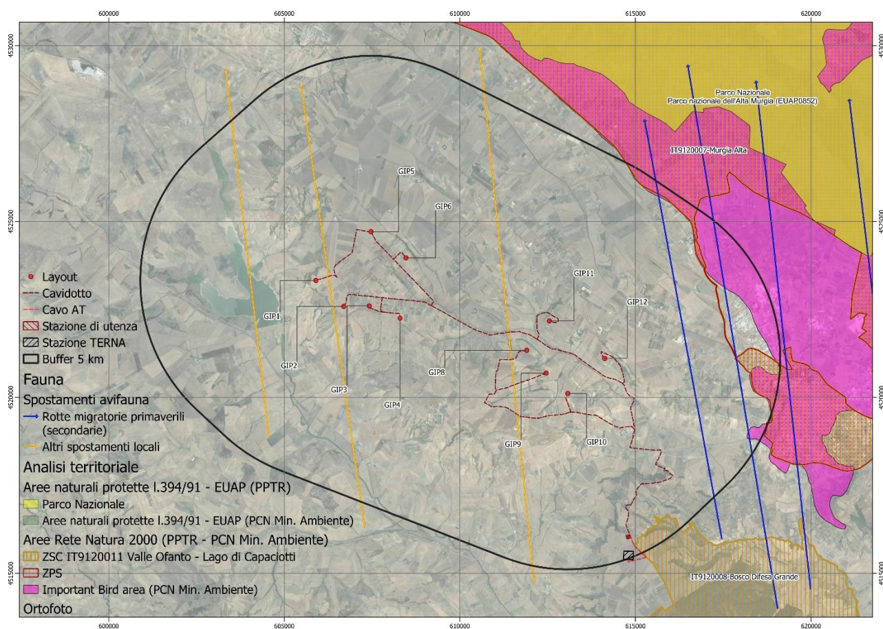
Figura 26: Rotte migratorie primaverili
