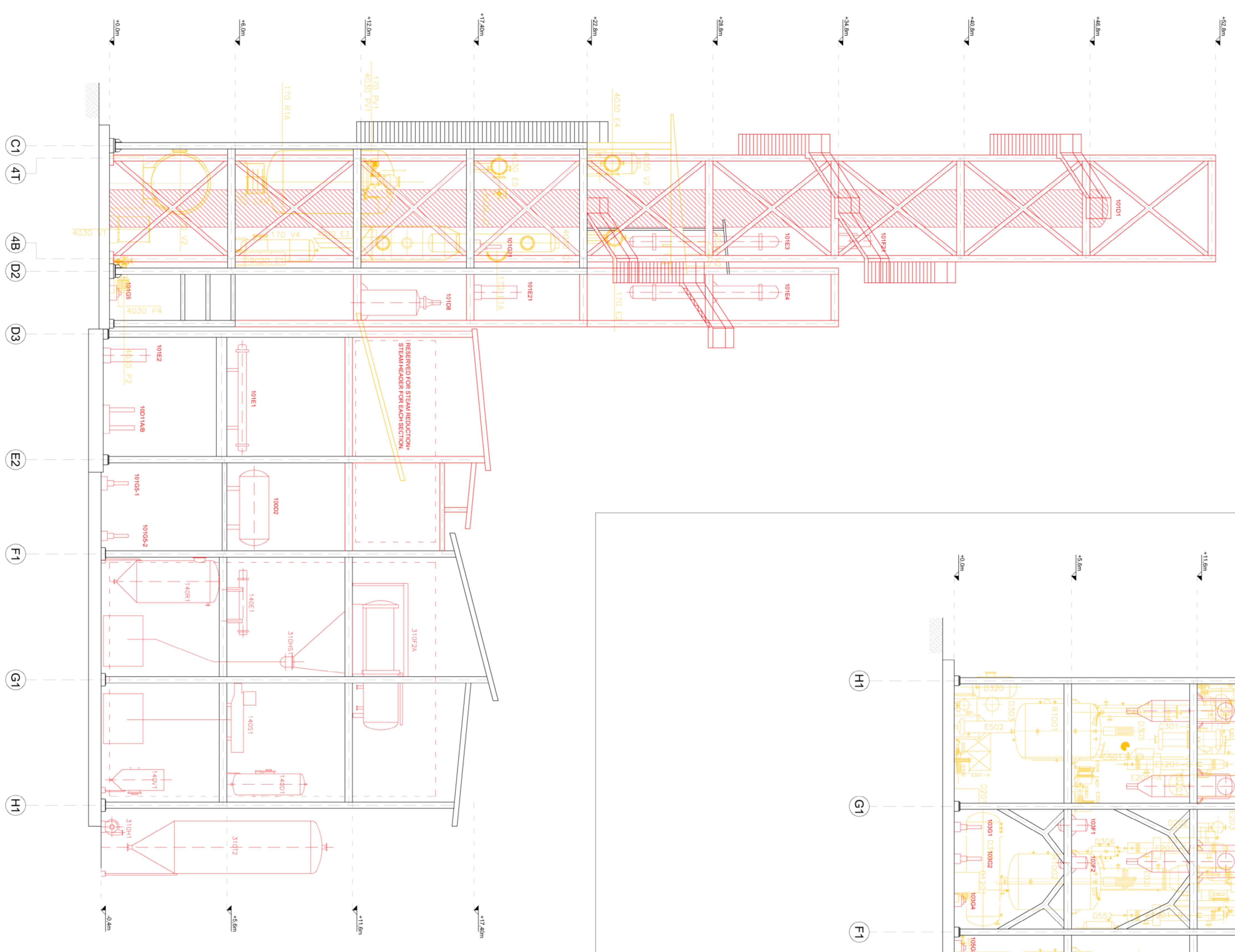
VISTA LATO SUD. SCALA 1:100
