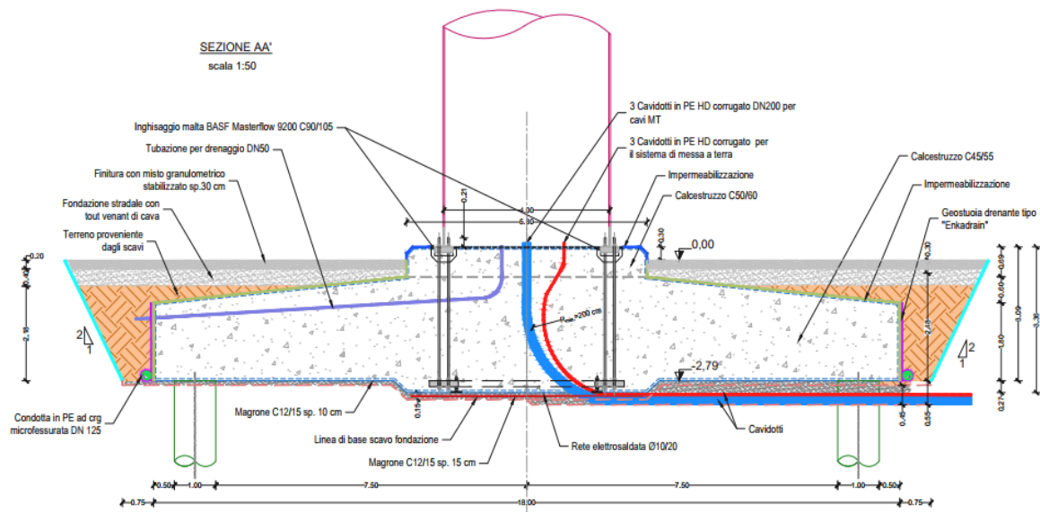
Fig.16 Sezione del plinto
