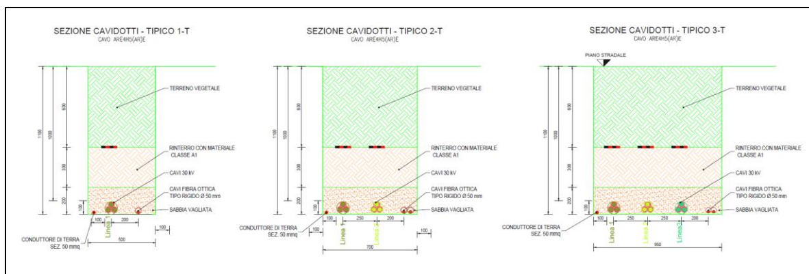
Fig. 25 – Sezioni tipo di scavo su terreno vegetale
