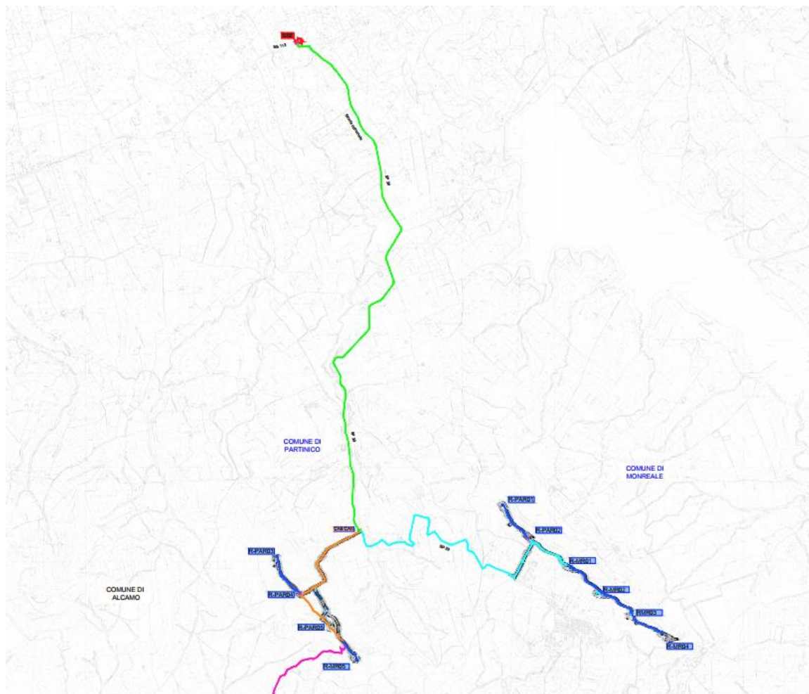
Fig.20 - Layout cavidotti su Carta regionale tecnica
