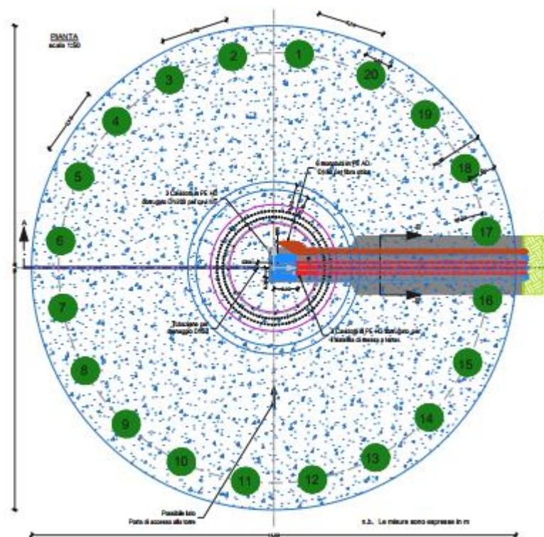
Fig.15 Pianta del plinto con indicazione dei pali di fondazione (n.20 del diametro 100 cm)
