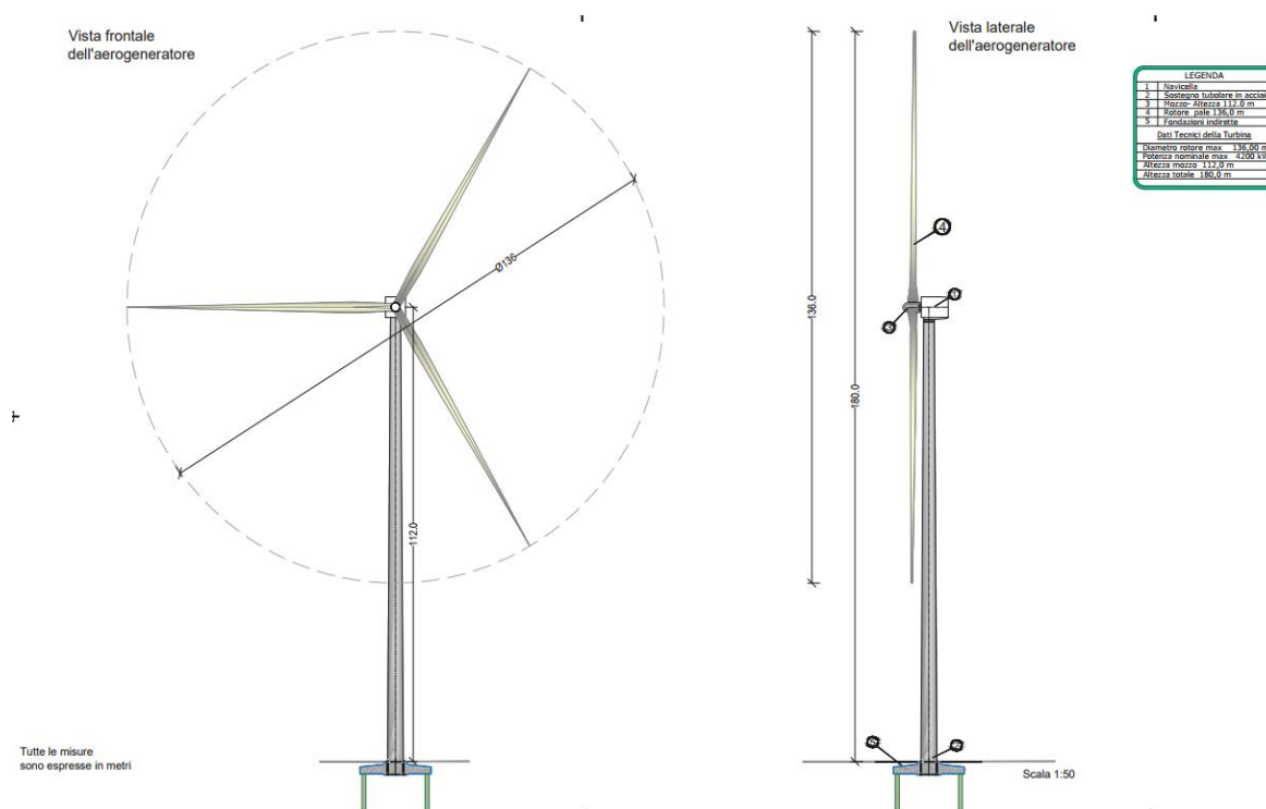
Fig.7 Schema tipo aerogeneratore
