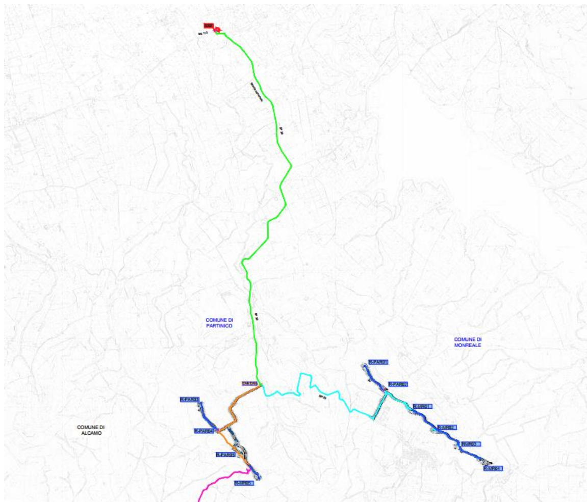
Fig.6- Inquadramento impianto su ctr 1:10.000
