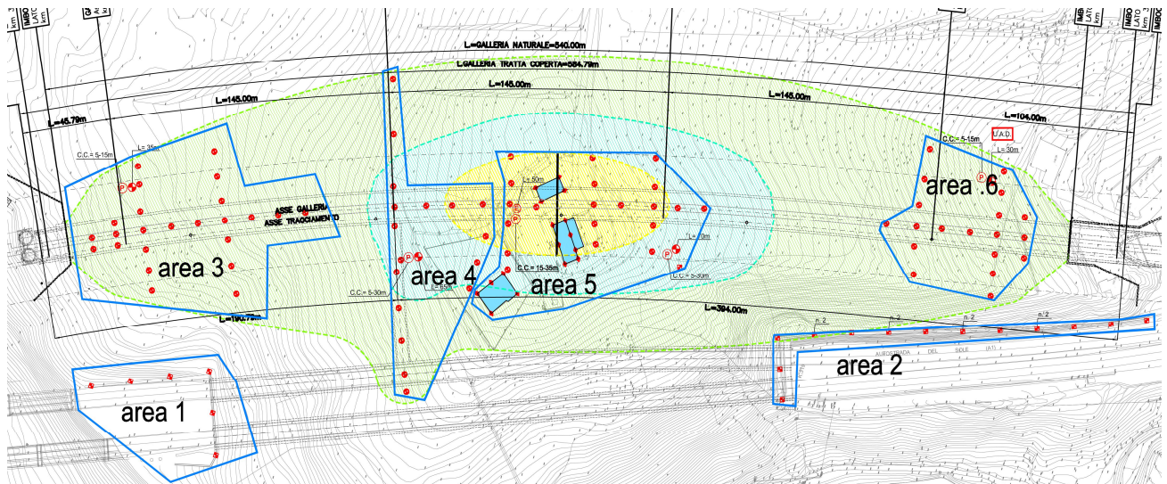
Figura 1: Siti di monitoraggio topografico per controllo subsidenza
