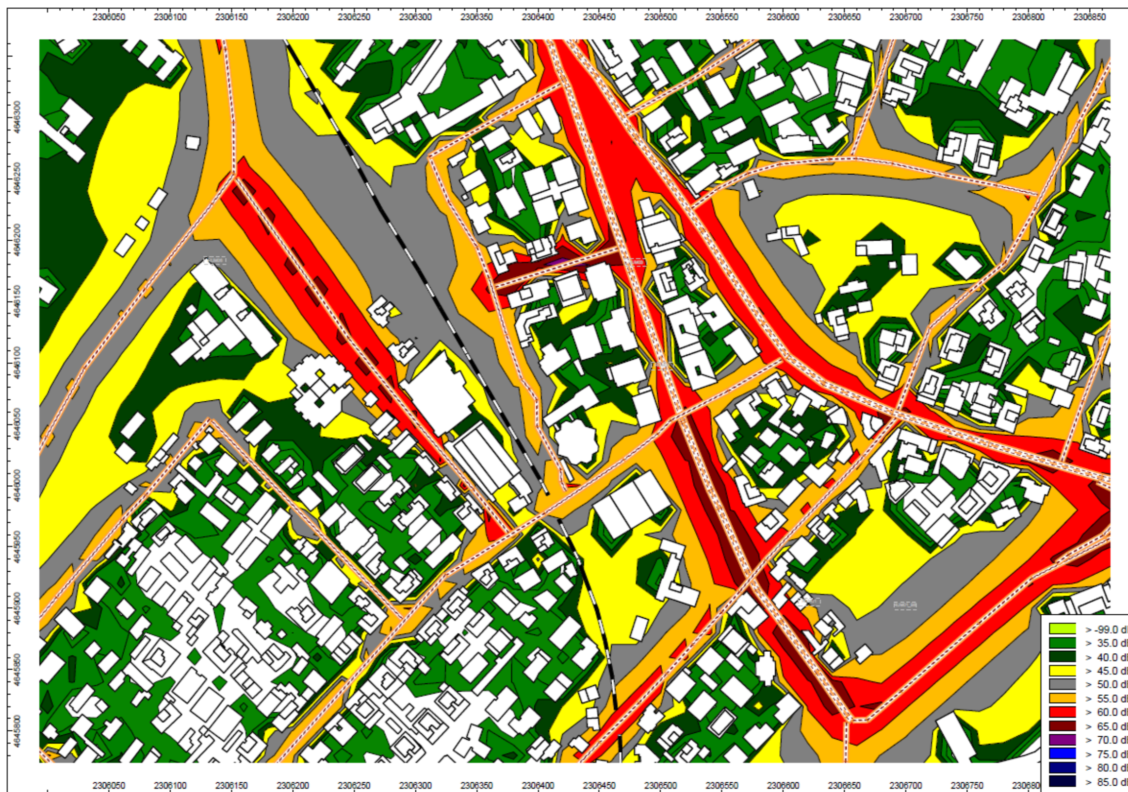
Figura 2-98 - - Isofoniche situazione attuale, periodo notturno.
