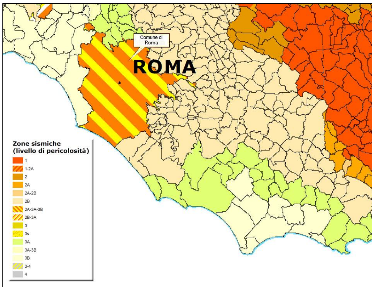
Figura 2-32 - Zone sismiche aggiornate dall'OPCM 3274/2003 e recepite dalle Regioni – Aggiornamento al 2021.
