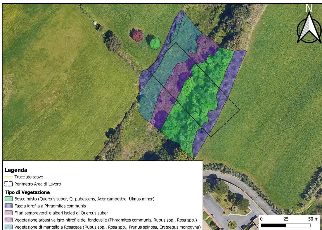
Figura 2-71 Inquadramento della vegetazione nei pressi dell'area di lavoro
