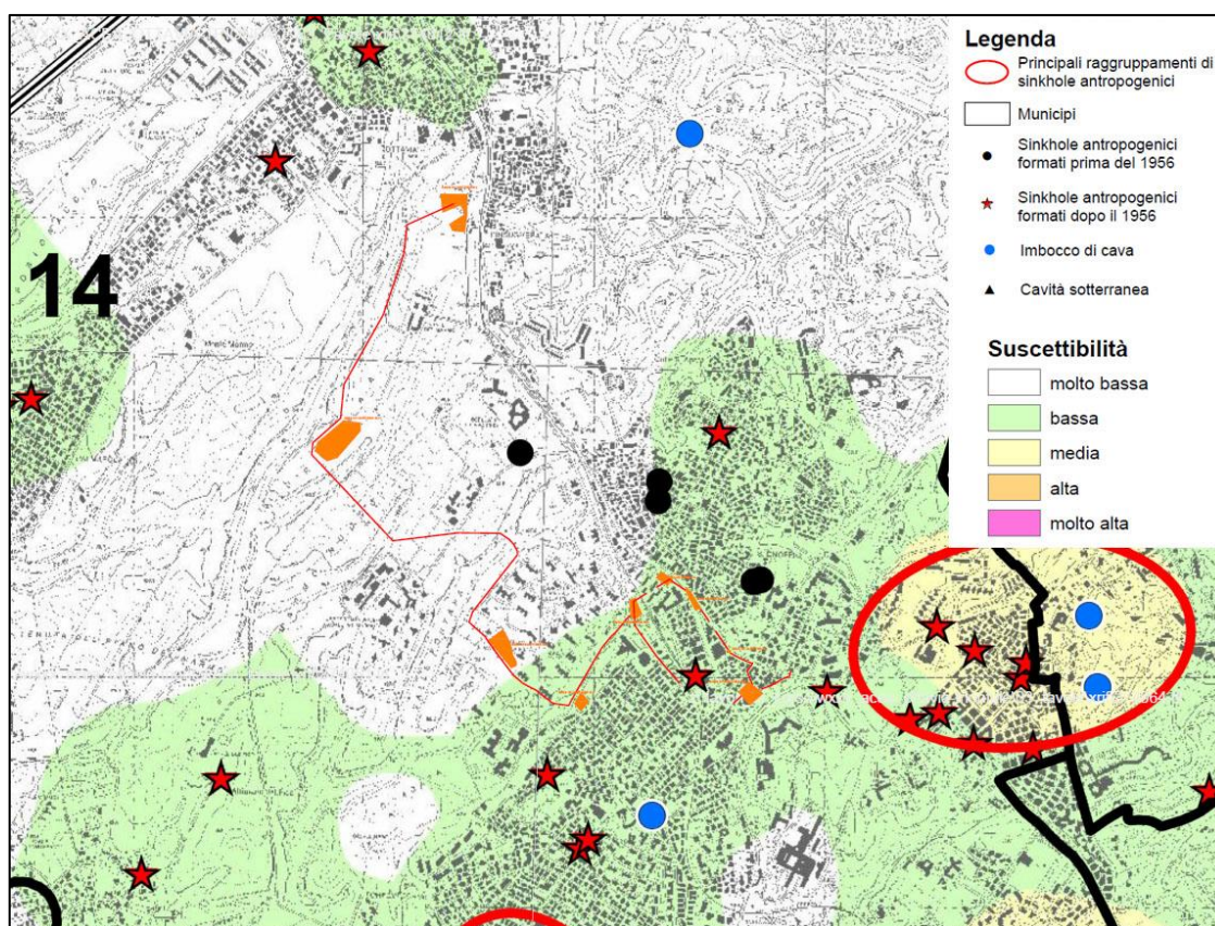
Figura 2-29 - Stralcio della Carta della Suscettibilità ai Sinkholes Antropogenici nel Centro Urbano di Roma (in rosso il progetto).
