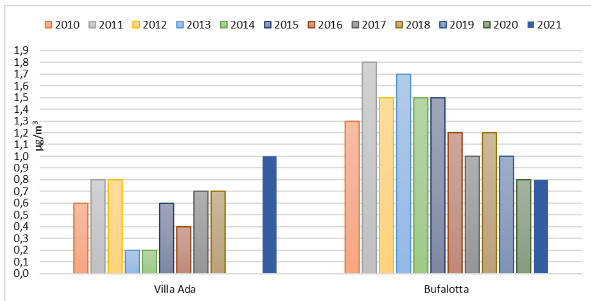
Figura 2-22 – Media Annua SO 2 , anni 2010-2021.
