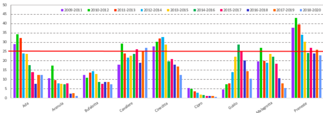
Figura 2-19 – Agglomerato di Roma - O 3 - superamenti 120 \mu\text{g}/\text{m}^3 (fonte Valutazione della Qualità dell’Aria della Regione Lazio 2020).
