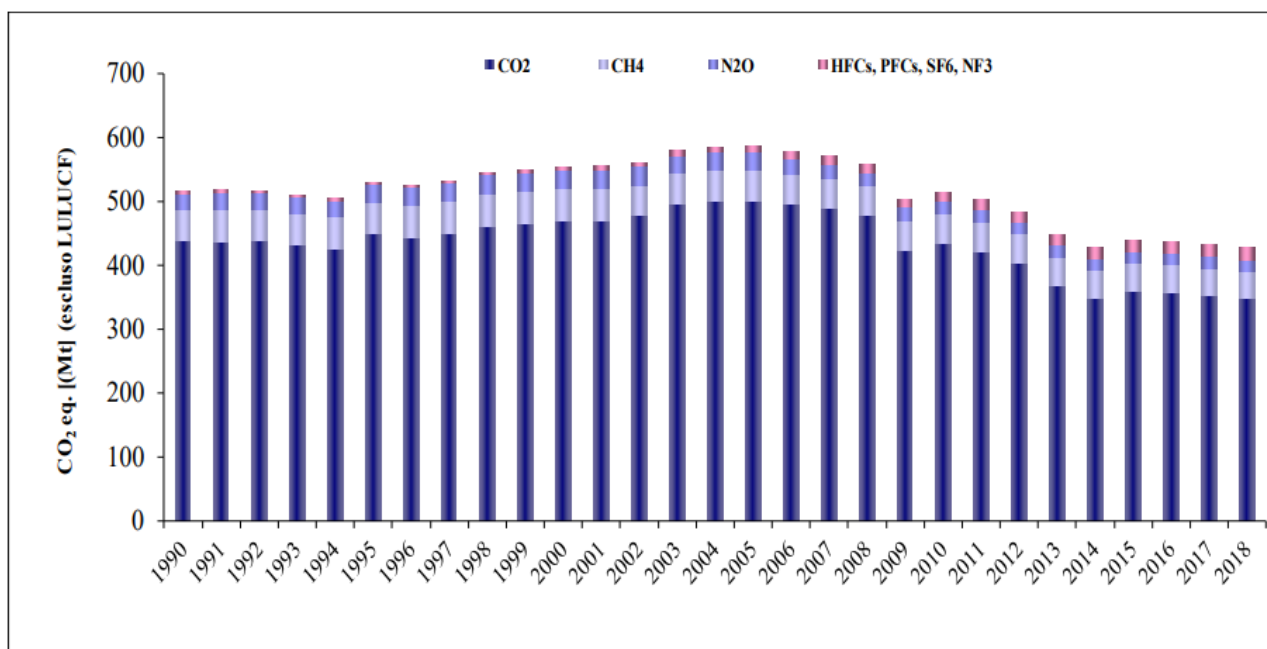
Figura 2-23 – Emissioni nazionali di Gas Serra suddivise per gas principali. Fonte: ISPRA.
