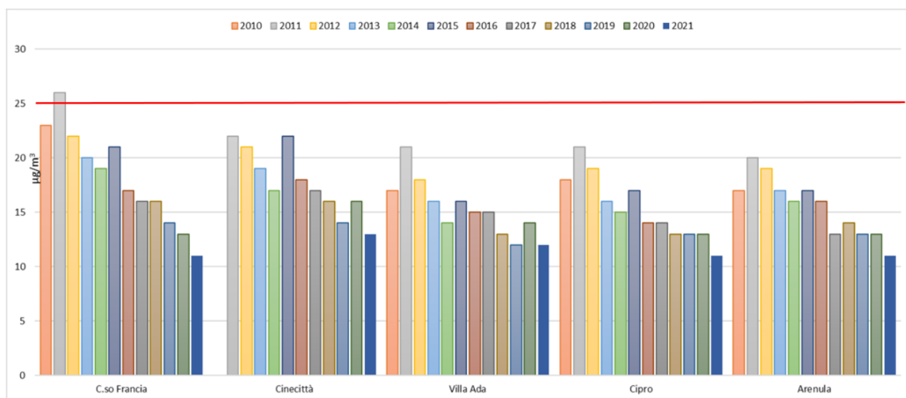
Figura 2-18 MEDIE ANNUE PM_{2,5} , anni 2010 – 2021 – Stazioni comprese nel GRA di Roma.
