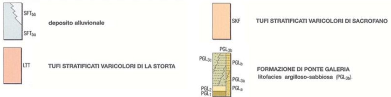
Figura 2-31 – Stralcio Carta geologica Progetto CARG –Foglio 374 ROMA (in blu il progetto)
