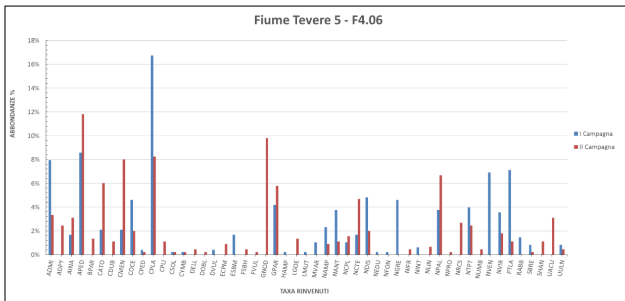
Figura 2-41 - Abbondanze percentuali dei taxa rinvenuti nei campioni delle due campagne di monitoraggio.
