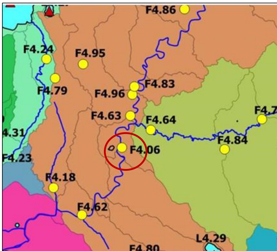
Figura 2-39 - Rete di monitoraggio della regione -Lazio (fonte-. https://sira.arpalazio.it/web/guest/corpi-idrici-e-reti-di-monitoraggio ). Nel riquadro rosso è indicato il punto preso come riferimento per la qualità delle acque superficiali.
