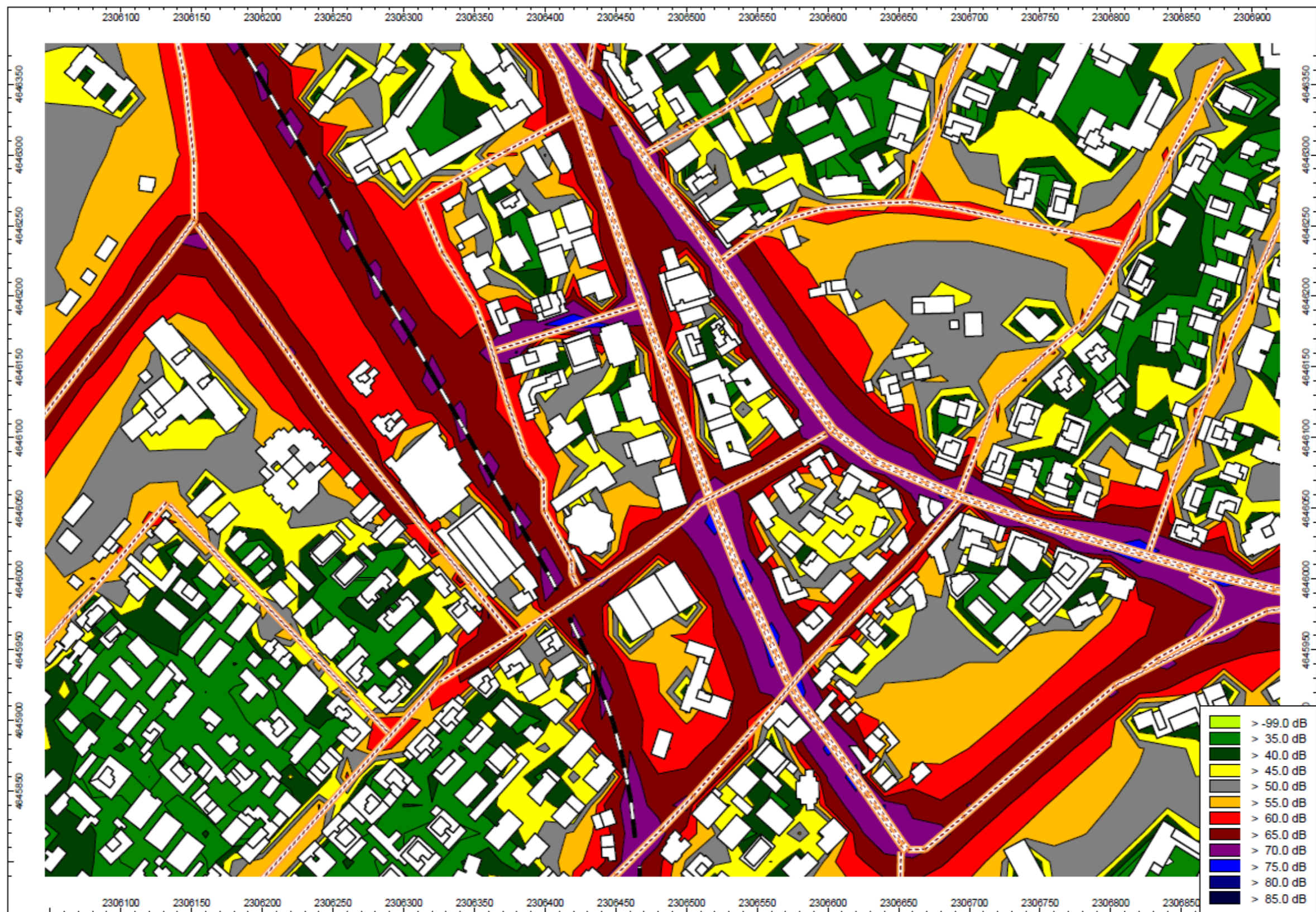
Figura 2-99 - Isofoniche situazione attuale considerando i transiti ferroviari, periodo diurno.
