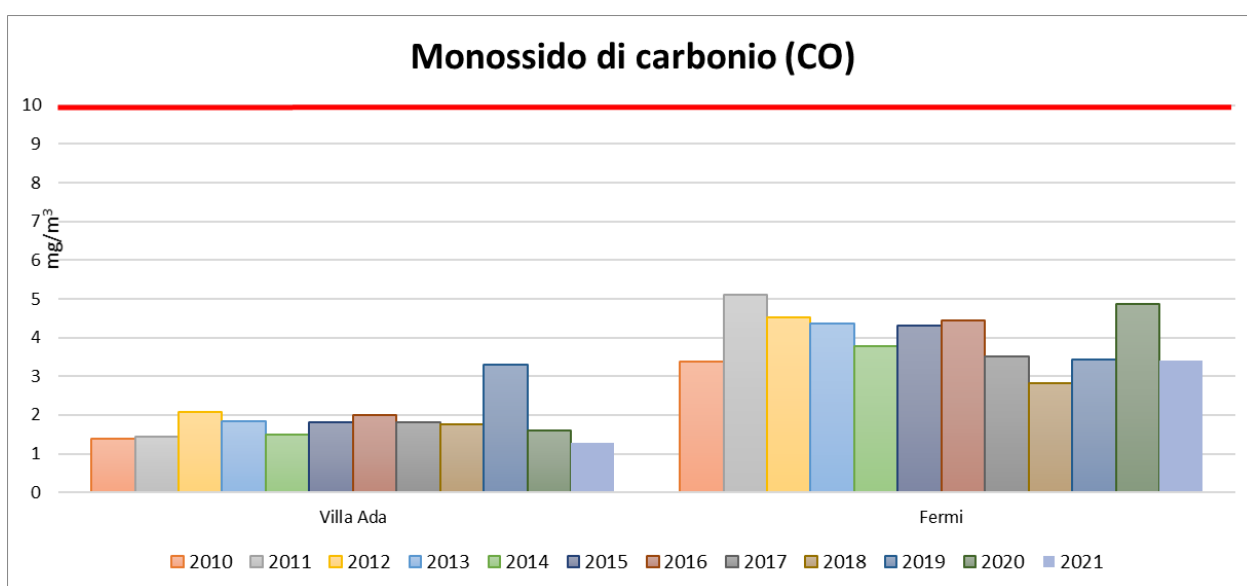
Figura 2-21 - Media massima giornaliera su 8 ore del CO, anni 2010-2021 – stazioni Villa Ada e Fermi.
