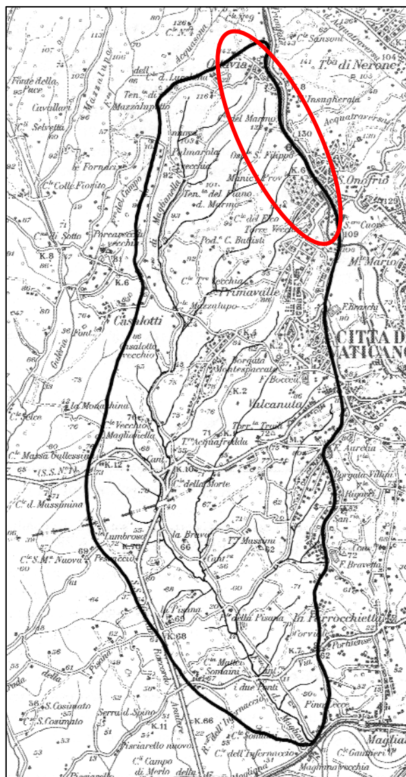
Figura 2-36 - Bacino del fosso della Magliana (in rosso è indicata l’area d’indagine).
