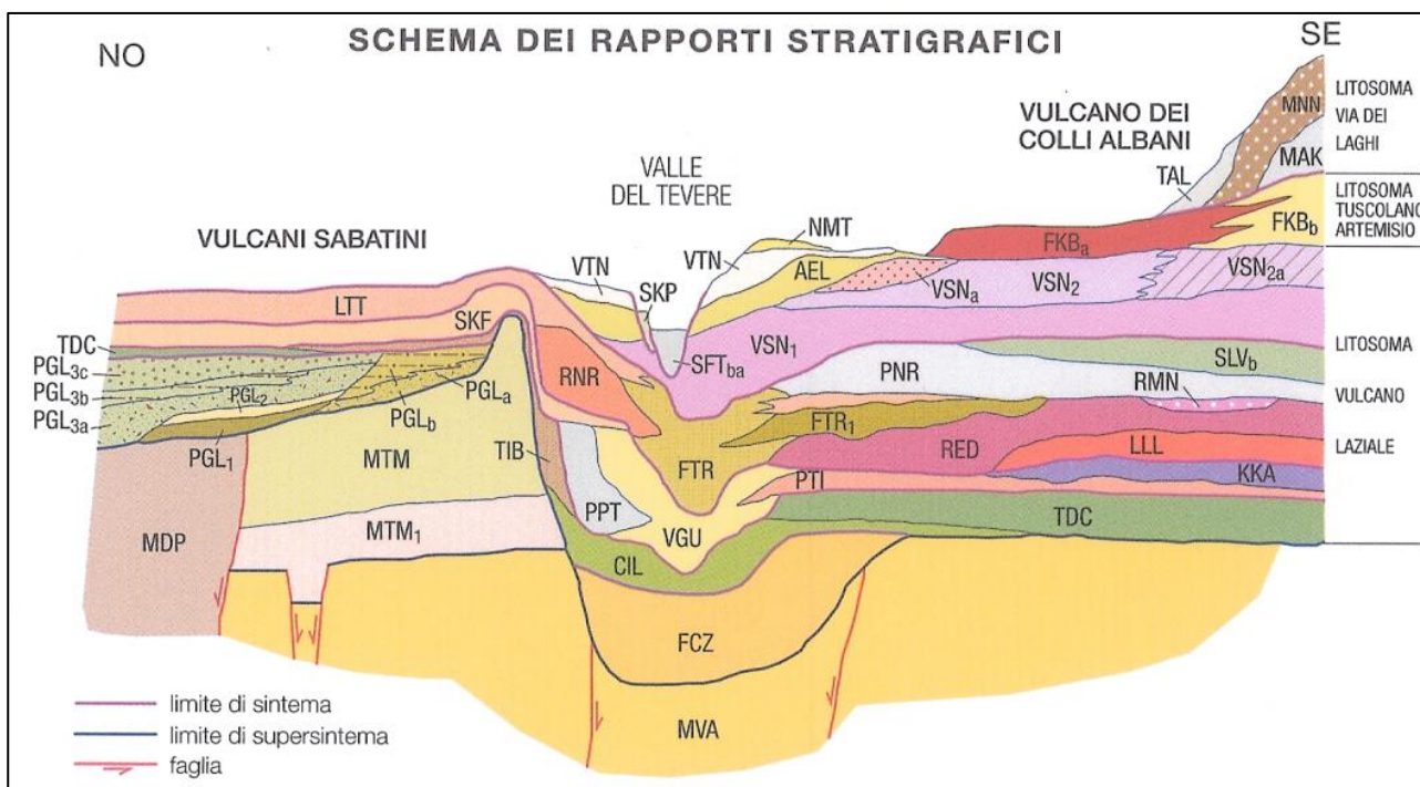
Figura 2-30 – Schema dei rapporti stratigrafici dell’area romana.
