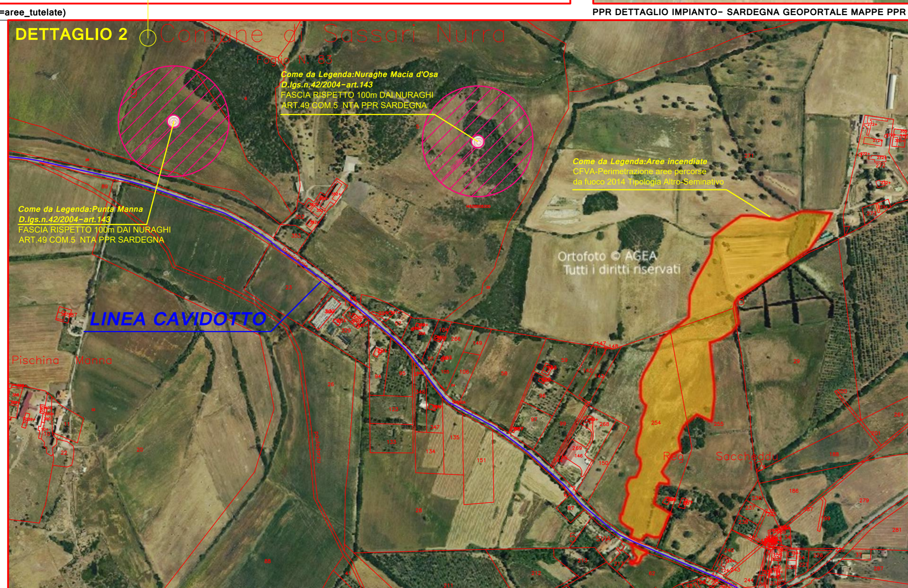
DETTAGLIO 2 CAVIDOTTO LUNGO BANCHINA SP 18 AREA NURAGHI PUNTA MANNA E MACCIA D'OSA CON SOVRAPPOSIZIONE E.D.M. N°83 CATASTALE SCALA 1:100
