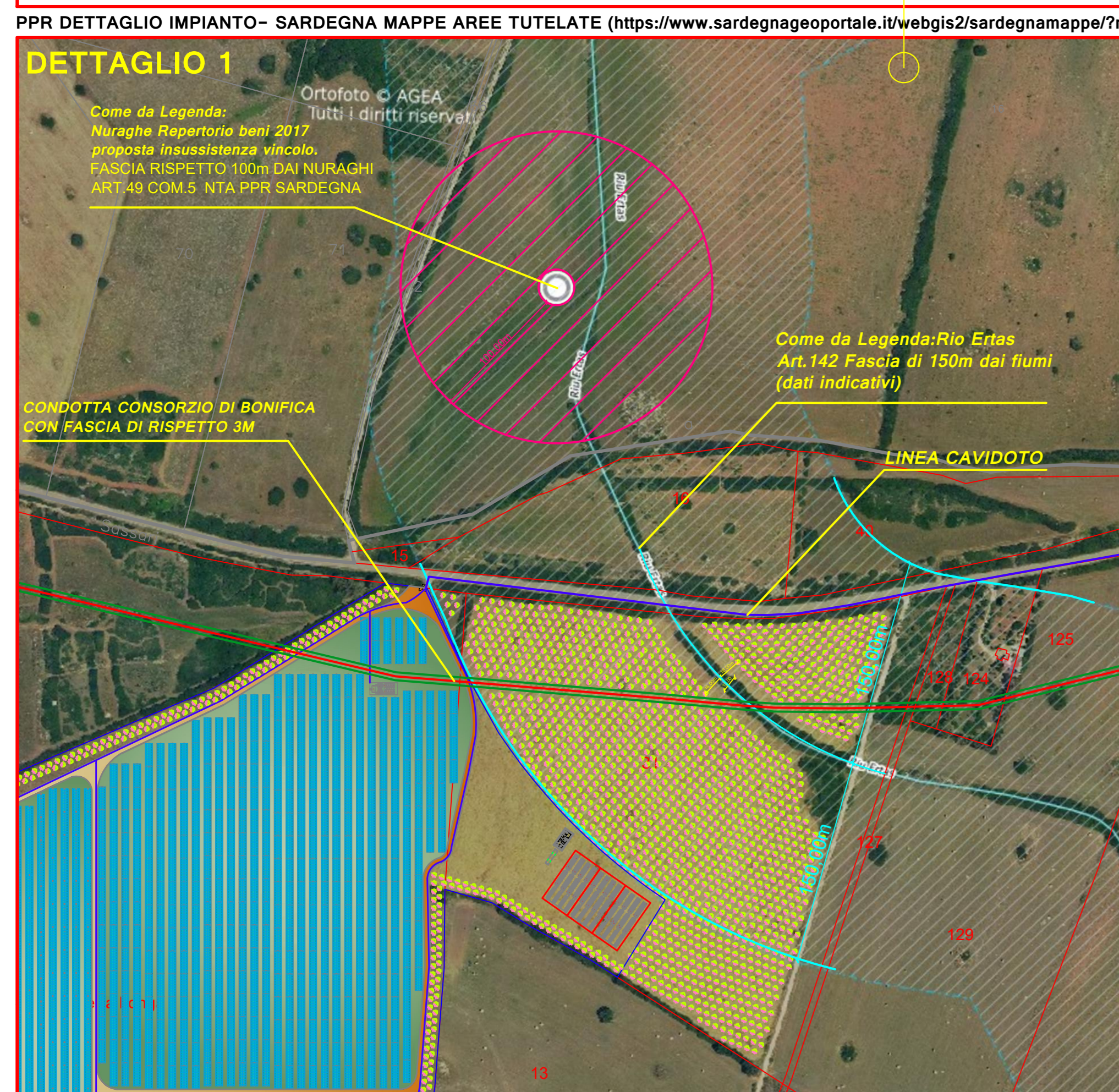
DETTAGLIO 1 IMPIANTO AREA MANDORLETO E RIO ERTAS CON SOVRAPPOSIZIONE E.D.M. N°81 CATASTALE SCALA 1:100
