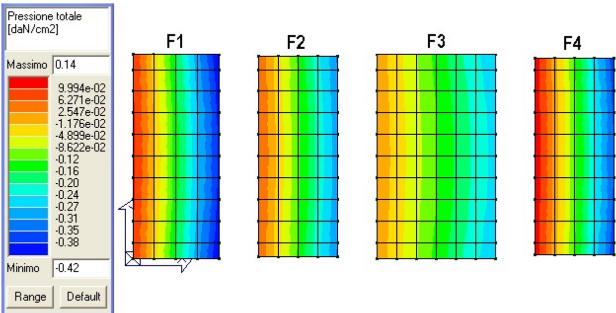
Mapa cromatica delle pressioni sul terreno - Comb. SLE freq.
