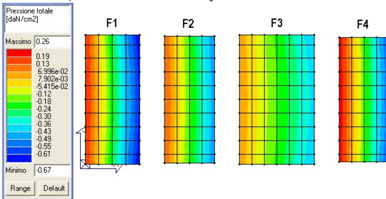
Mapa cromatica delle pressioni sul terreno - Comb. SLU
