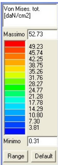
Mappa cromatica delle tensioni totali (membrana + flessione) ottenute mediante la formulazione di Von Mises - Comb. SLE q. perm.
