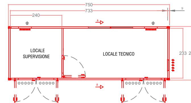
PIANTA
