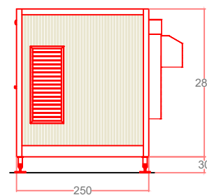
PROSPETTO SINISTRO
