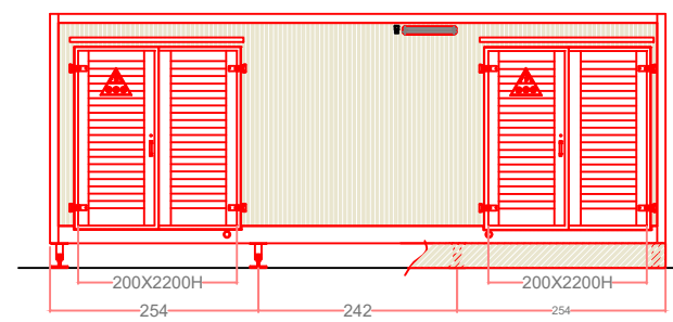
PROSPETTO ANTERIORE
