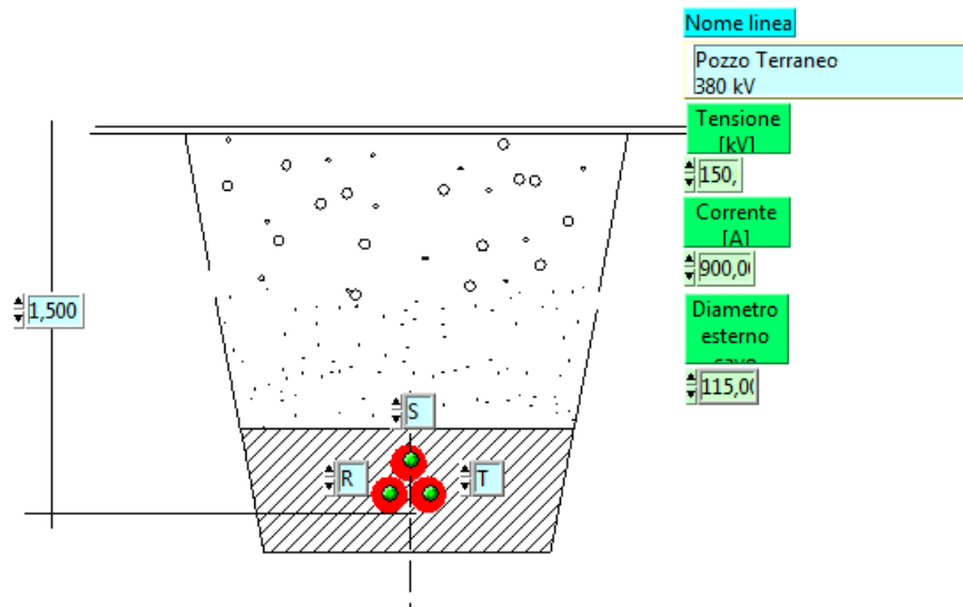
Figura 5 - Sezione tipo
