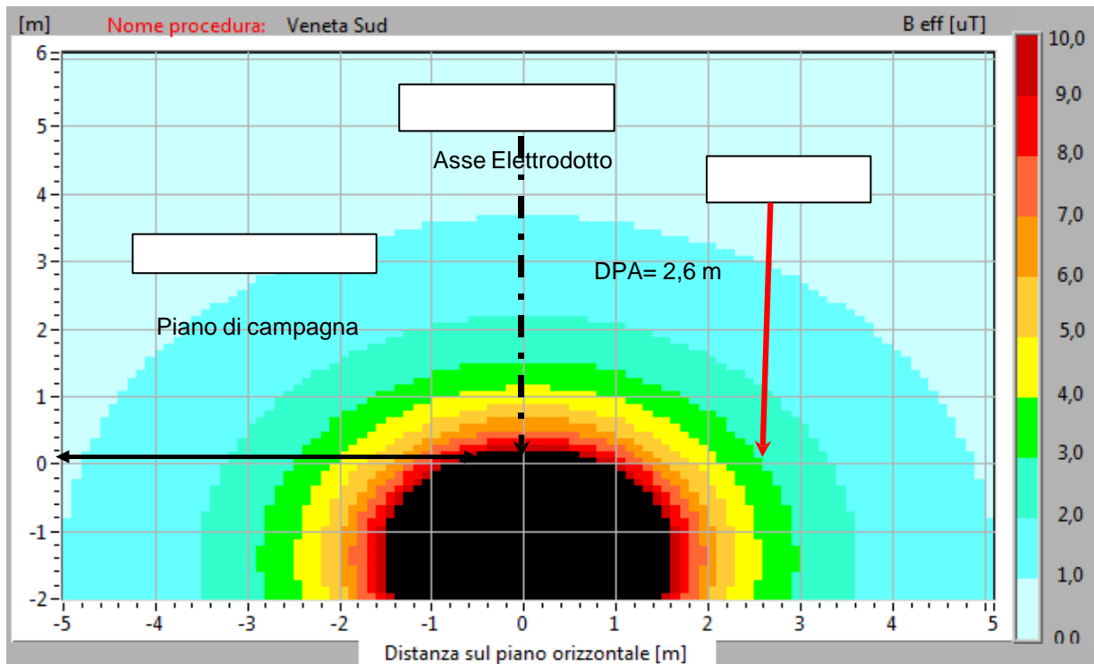
Figura 6 - Mappa verticale induzione magnetica (B) sezione tipo con indicazione della DPA - V=150 kV I= 900 A
