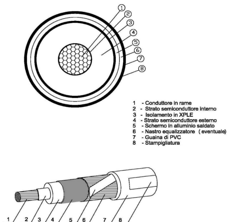
Figura 4 - Schema tipo cavo 150 kV
