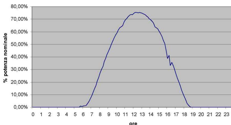
Figura 3 – Esempio del profilo di produzione per il 21 giugno (giornata serena)
