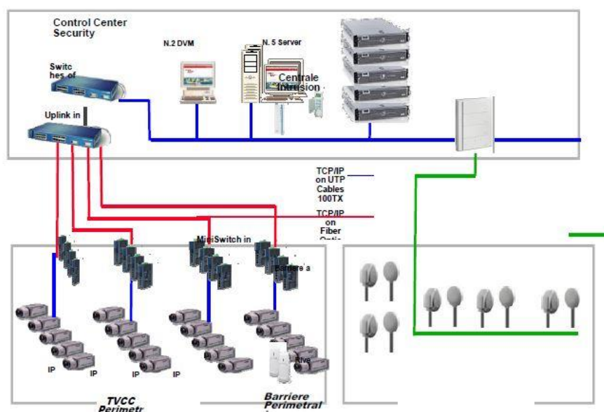
Figura 5 - Schema del sistema di videosorveglianza
