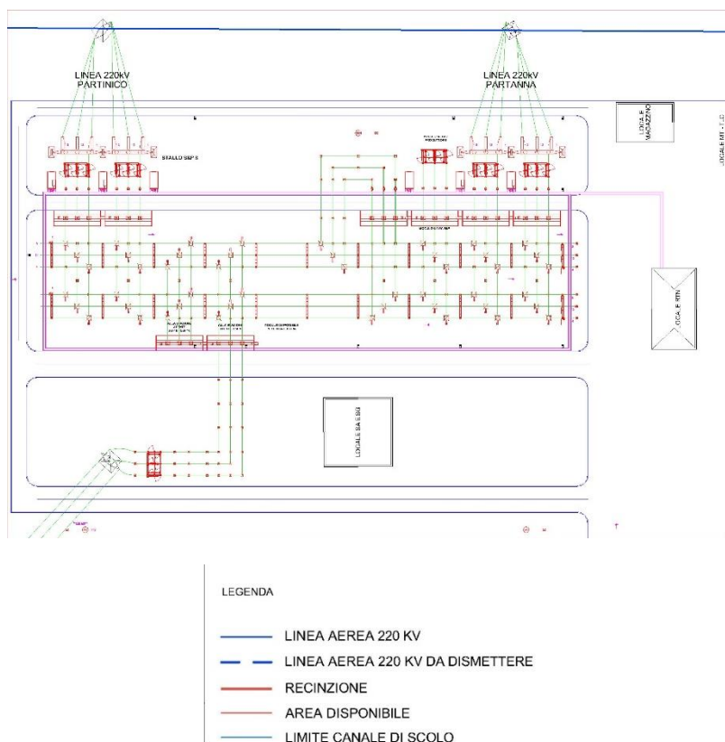
Figura 3 – Pianta elettromeccanica generale - Rete
