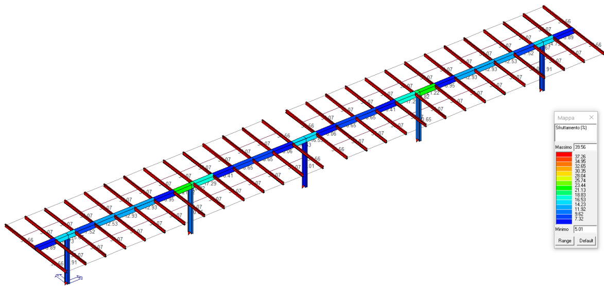
Figura 2 Verifica e Sfruttamento degli elementi Strutturali
