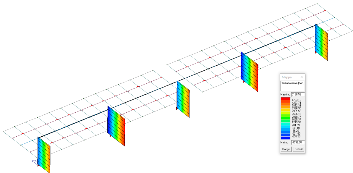
Figura 3 Diagramma degli sforzi normali
