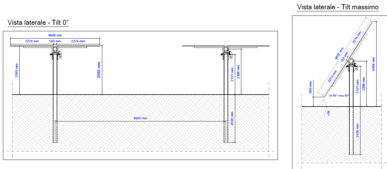
Figura 11: Caratteristiche dimensionali della struttura
