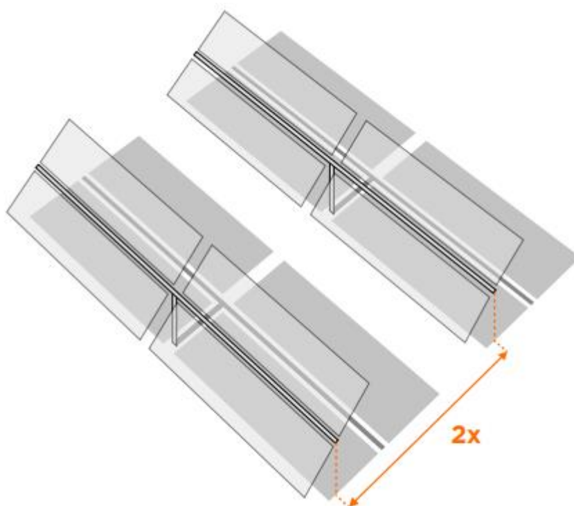
Figura 8: Esempio di installazione e ombre portate
