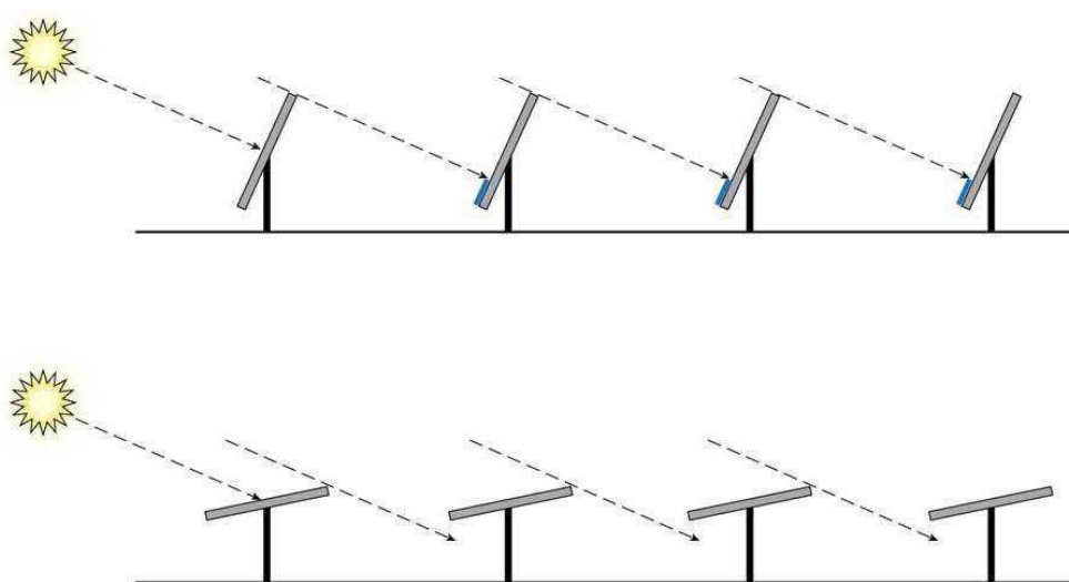
Figura 6: Rappresentazione del meccanismo di funzionamento della struttura
