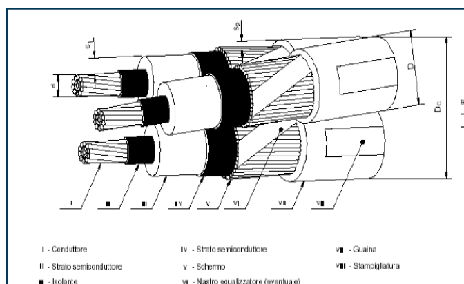
Figura 12: Cavo collegamenti MT
