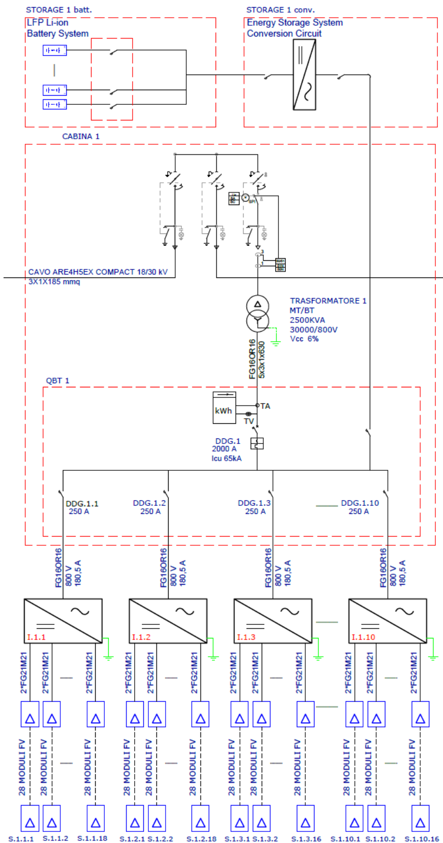
Figura 14: Schema unifilare collegamento Generatore-Trasformatore MT/BT
