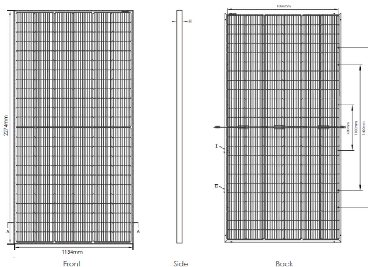
Figura 4 – Modulo fotovoltaico
