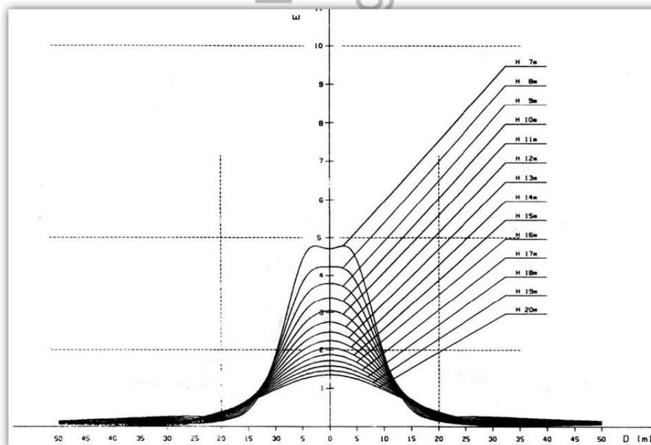
Fig. 2. Andamento tipico del campo di induzione magnetica.
