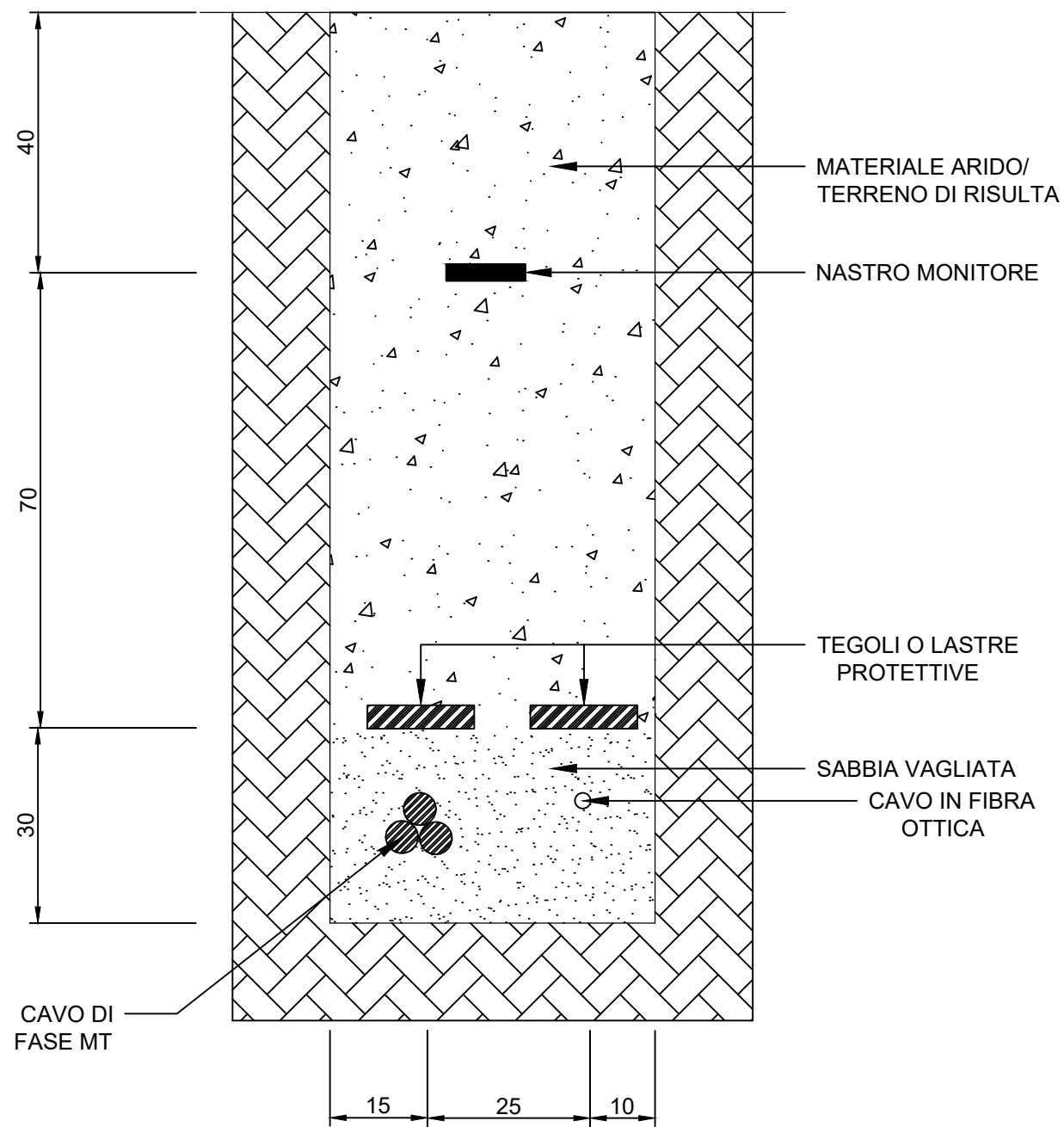
Sezione tipica di posa della linea MT in cavo in semplice trincea su strade sterrate.
