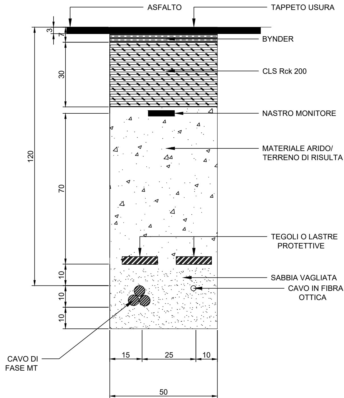
Sezione tipica di posa della linea MT in cavo in semplice trincea su sede stradale.
