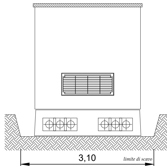
PROSPETTO D
