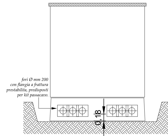
PROSPETTO C
