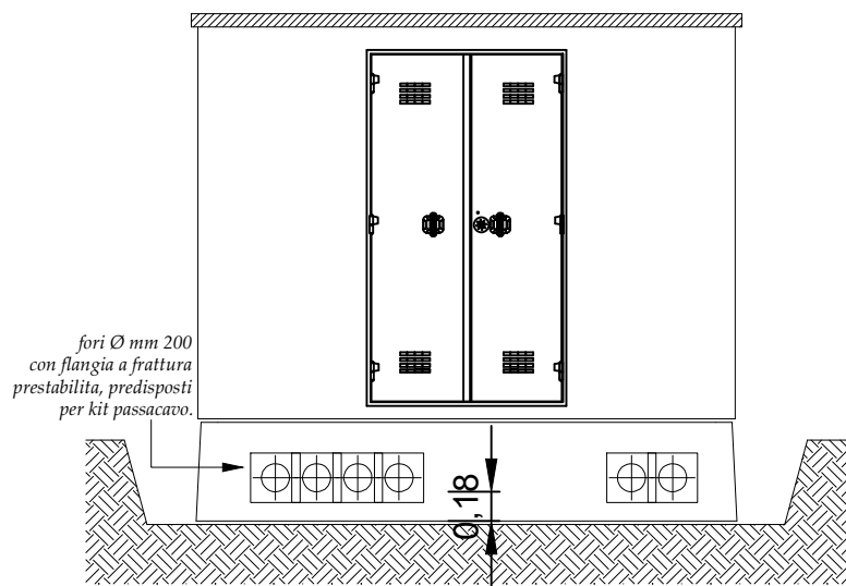
PROSPETTO A
