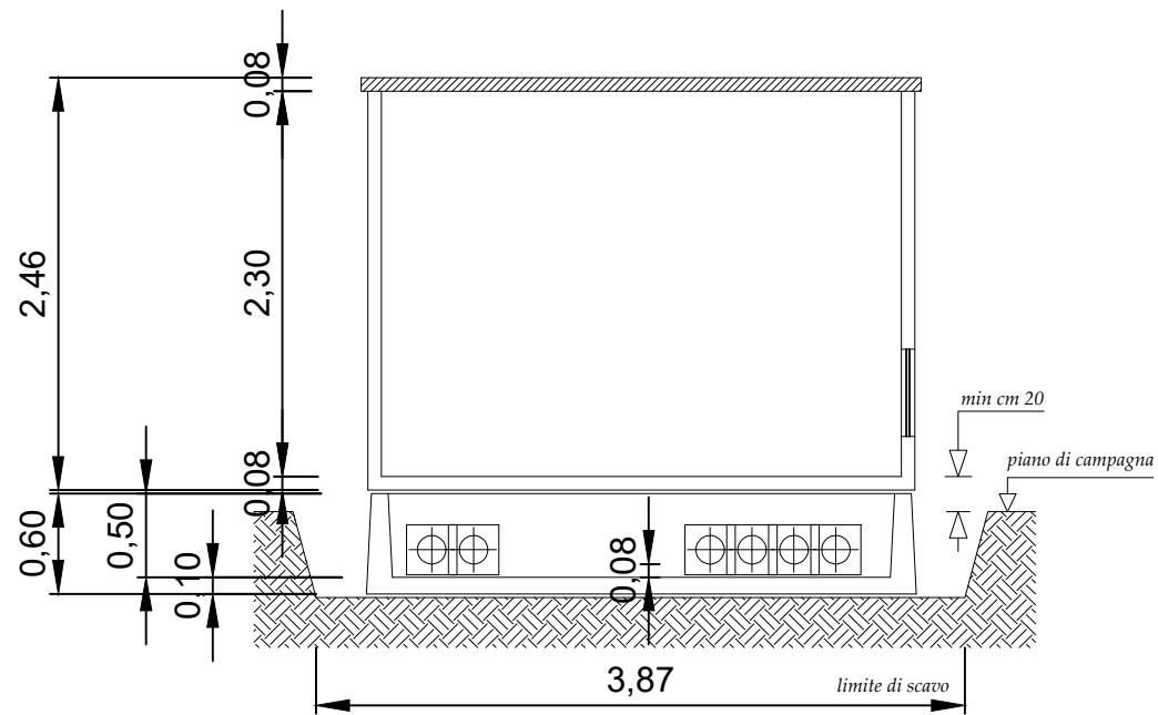
SEZIONE X-X
