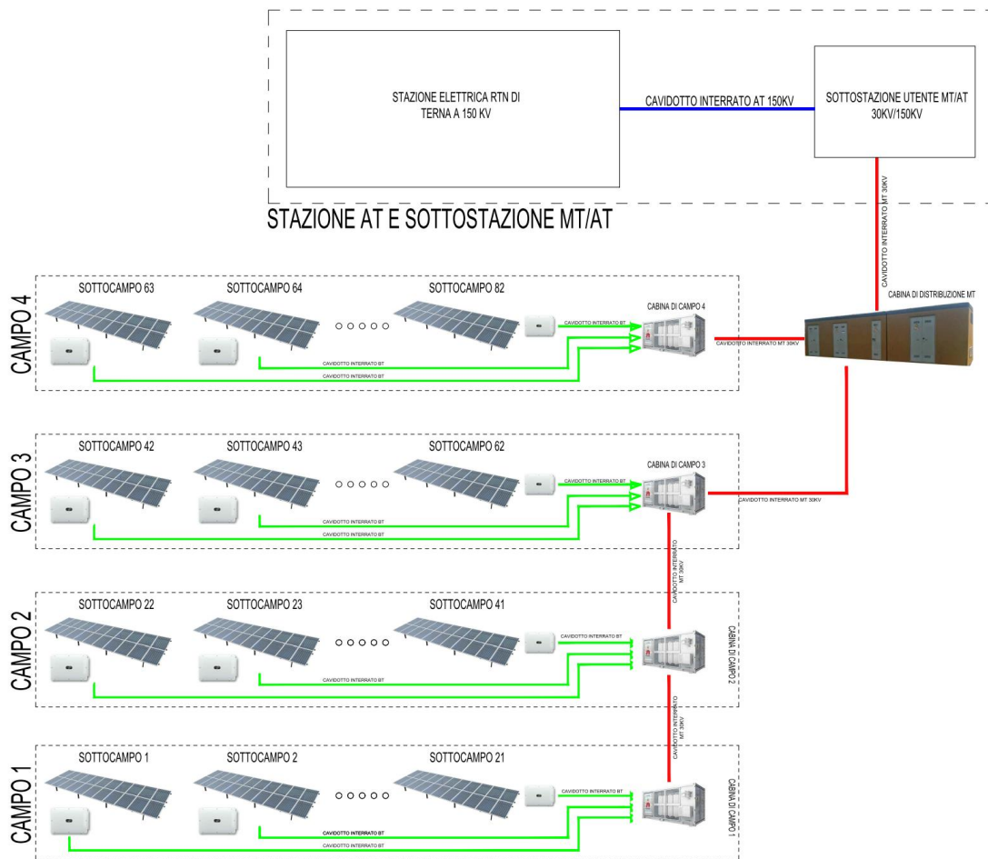
Figura 59 - Schema delle connessioni elettriche
