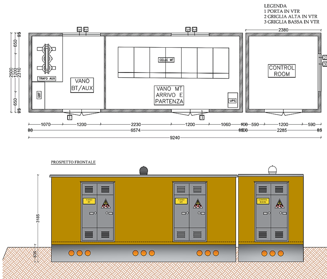
Figura 53 - Cabine
