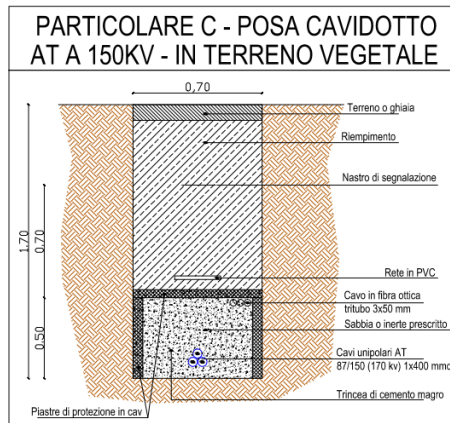
Figura 60 - Sezioni di scavo dei cavidotti
