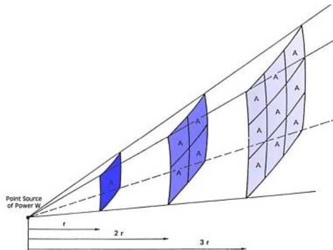
Figura 119 - divergenza geometrica (Fonte: www.slidetoDoc.com )
