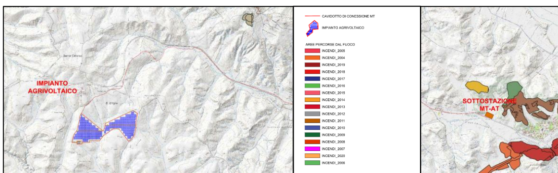
Figura 13 - Aree percorse dal fuoco
