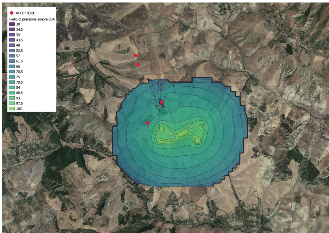
Figura 121 - Abstract del calcolo della diffusione della pressione sonora sulle aree limitrofe al cantiere in base ai dati di emissioni derivanti dalle macchine di cantiere (Fonte: ns elaborazione)
