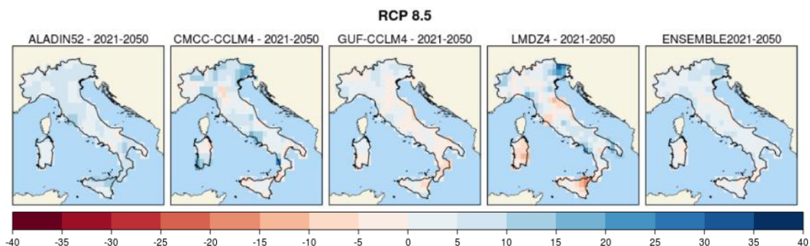
Figura 82 - Variazione dei totali di precipitazione giornalieri (mm), scenario RCP8.5(fonte: ISPRA)
