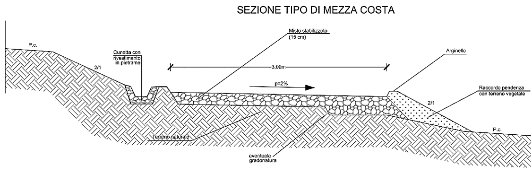
Figura 57 - Sezione tipo strade interne al sito, tipologia a mezza costa (Fonte: ns elaborazione)
