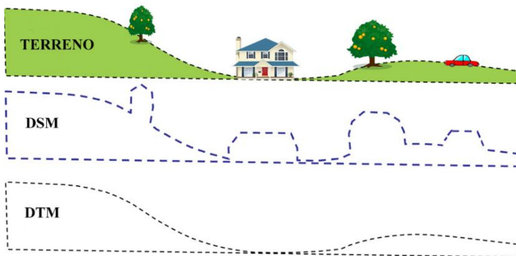
Figura 126 - Differenza tra DTM e DSM (6)
