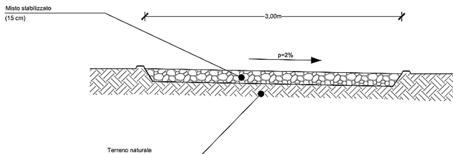
Figura 56 - Sezione tipo strade interne al sito di progetto (Fonte: ns elaborazione)
