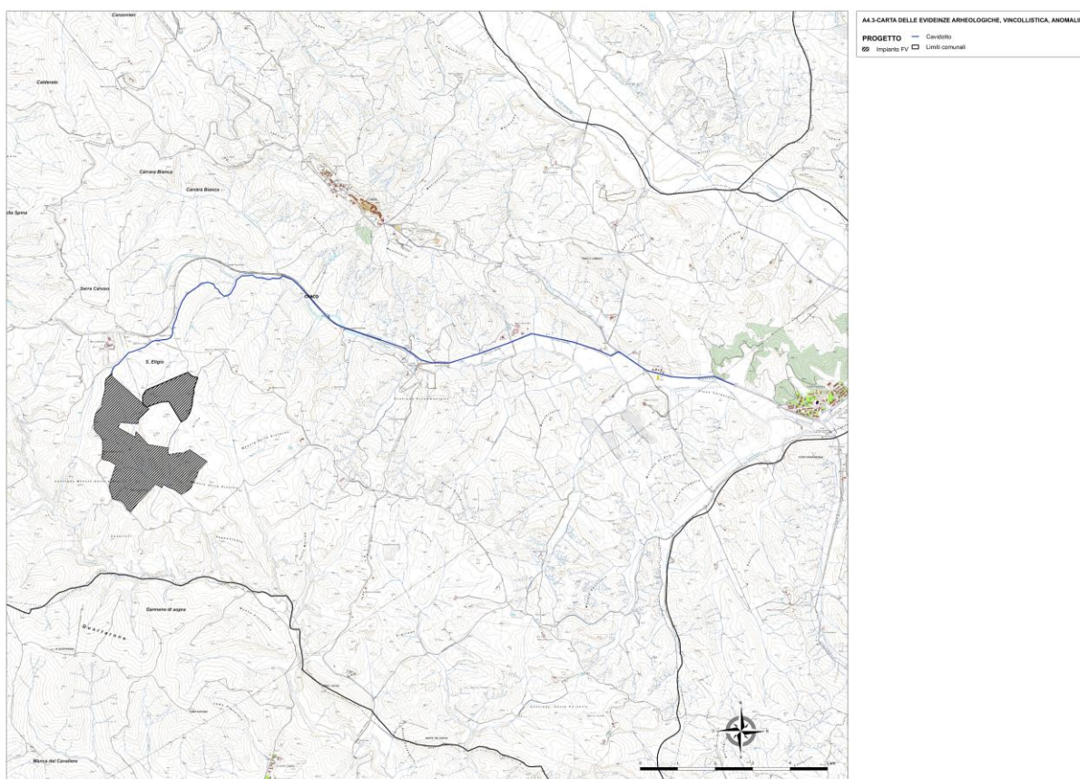
Fig. 1 – Planimetria generale dell'impianto fotovoltaico base CTR
