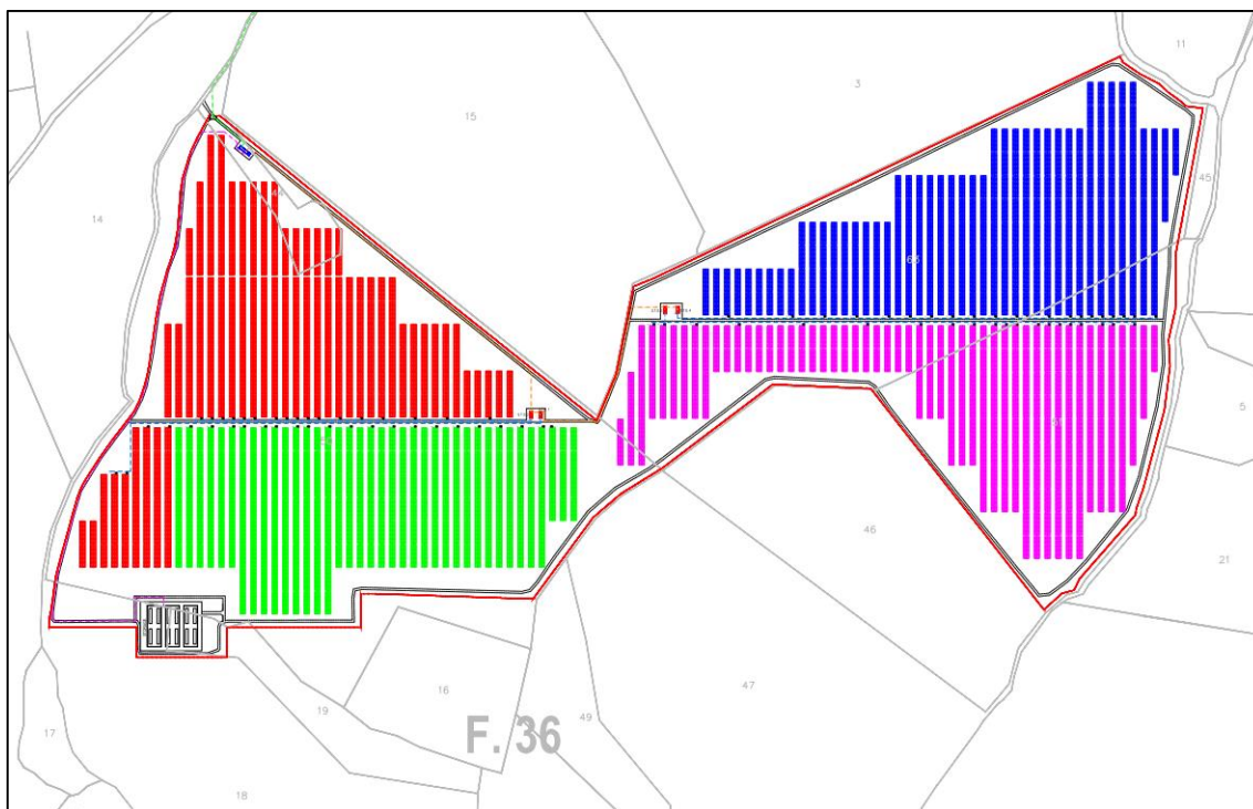
Figura 1 - Planimetria impianto agrivoltaico
