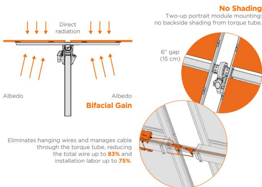
Figura 4 - Dettagli tacker
