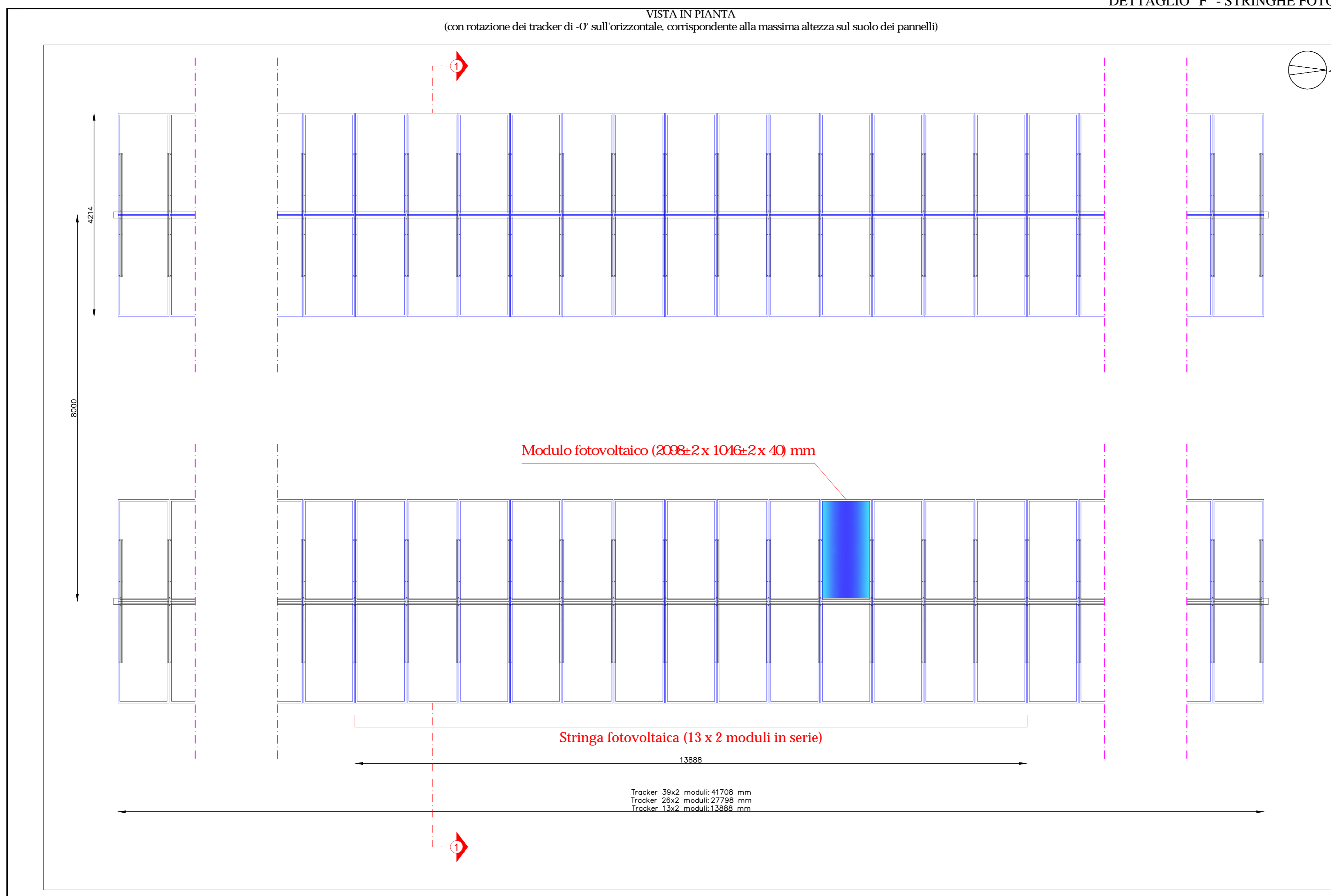
DETTAGLIO - TRACKER - scala 1:25 (quote in millimetri)
