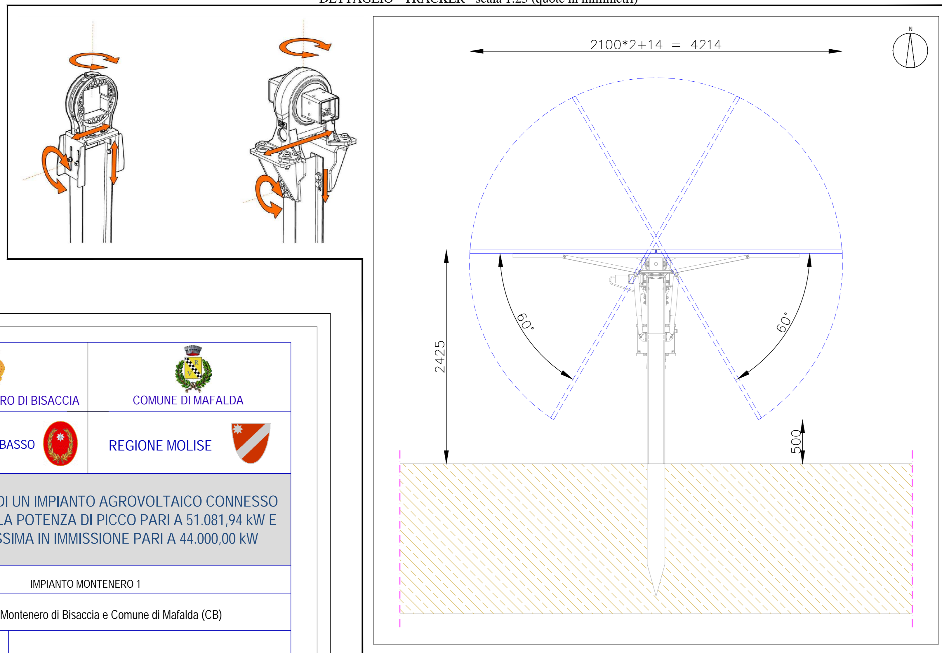
DETTAGLIO - TRACKER - scala 1:25 (quote in millimetri)
