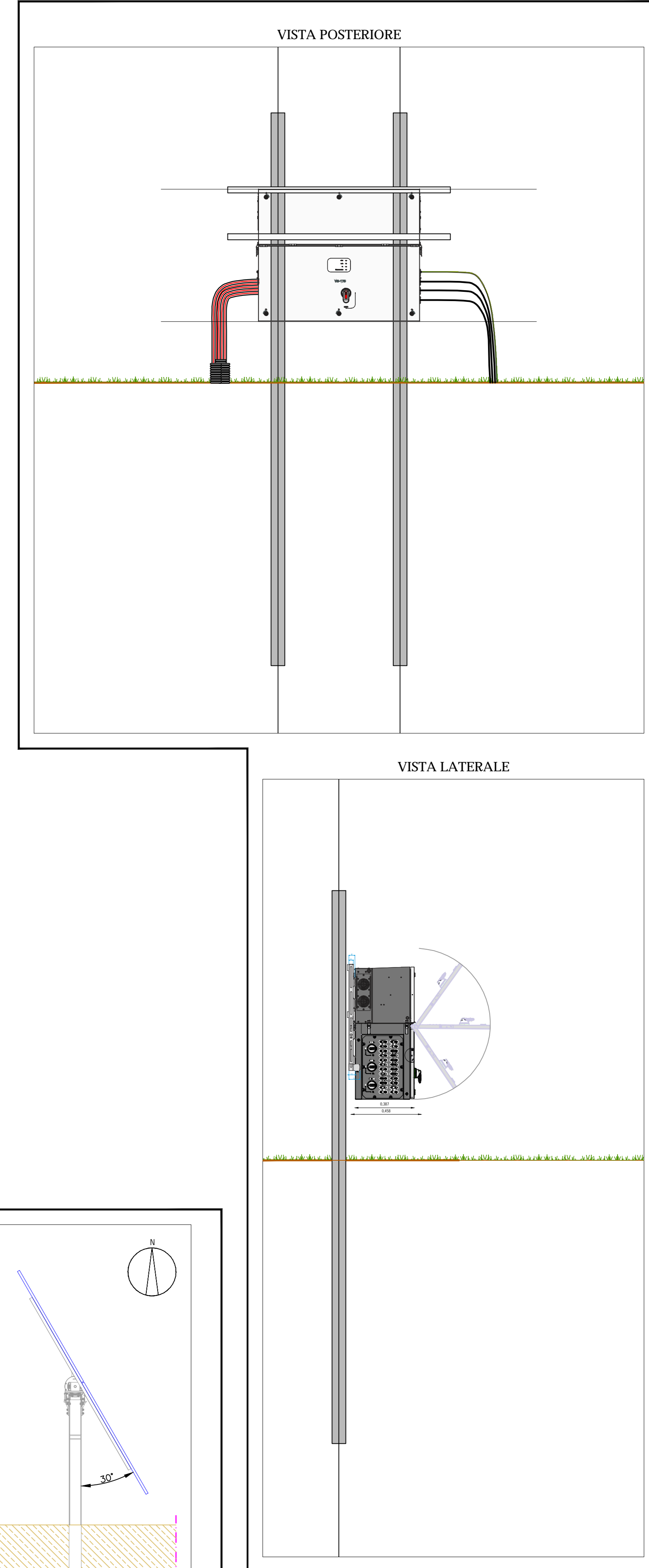
DETTAGLIO - INVERTER DI STRINGA - scala 1:20
