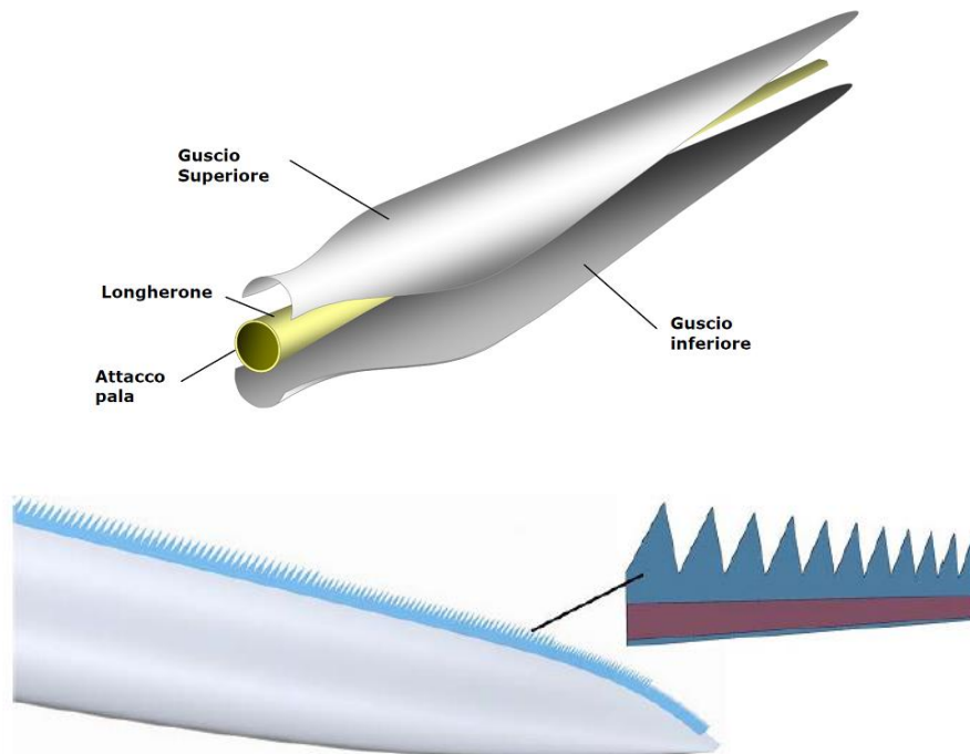
Figura 7 Particolare costruttivo della pala e delle dentellature (opzionali) di ottimizzazione del livello di rumore
