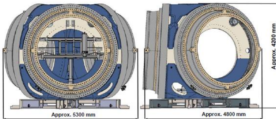
Figura 10 Mozzo (Hub)
