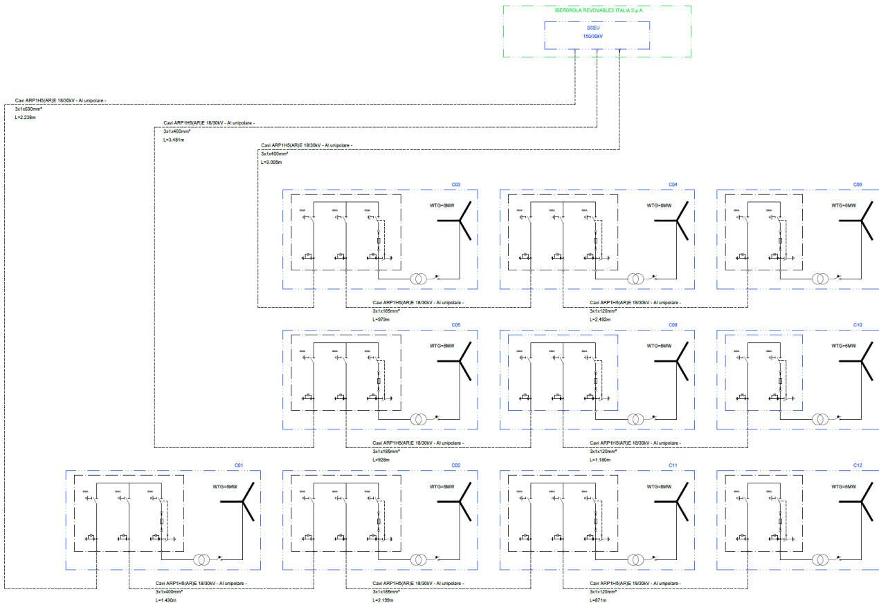
Figura 12 Schema elettrico unifilare MT aerogeneratori di progetto
