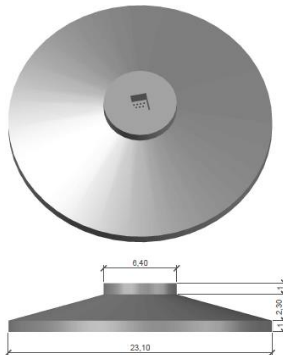
Figura 1 Fondazione Tipo
