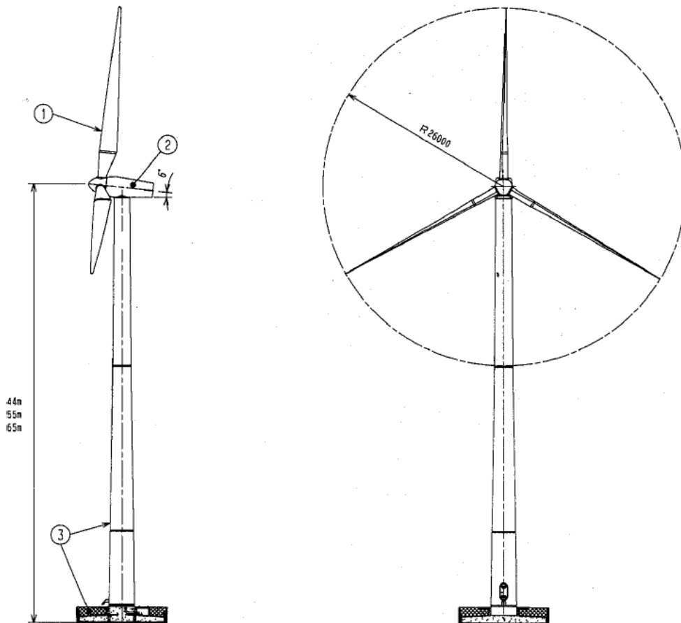
Figura 3-4: Dimensioni principali di una Gamesa G52
