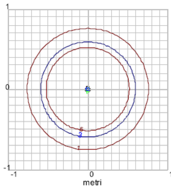
Figura 4: Curve di equilivello per il campo magnetico di una linea MT in cavo elicordato interrato (dalla Norma CEI 106-11)
