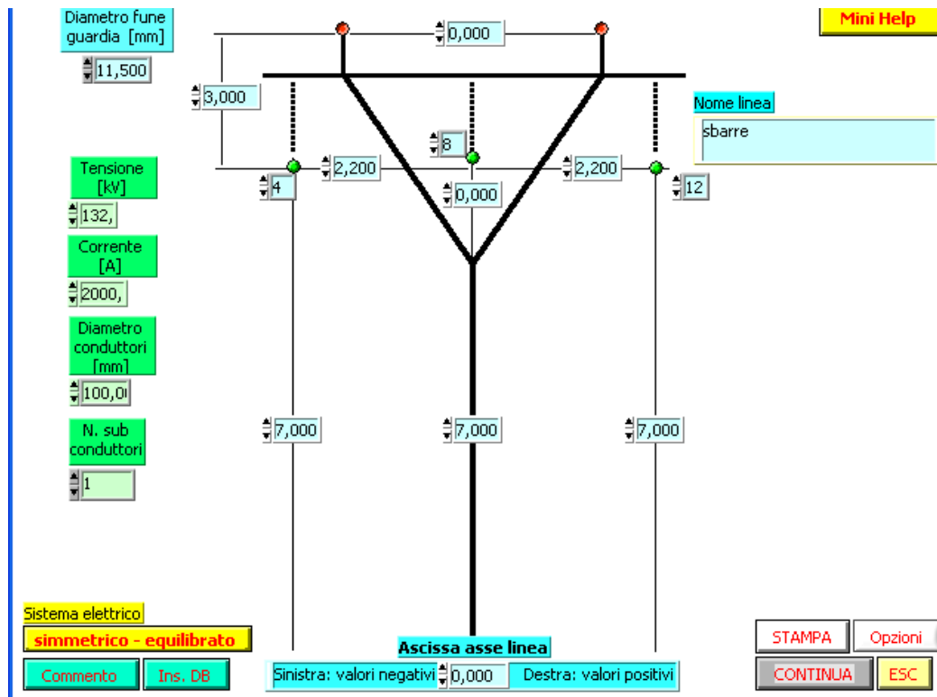
Figura 11: Linea AT con disposizione conduttori in piano assimilabile ad un sistema semplice sbarra a 220 kV.
