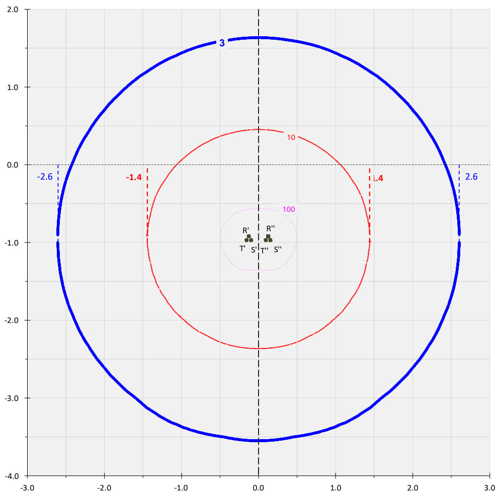
Figura 9: Curve di equilivello per il campo di induzione magnetica generato da una linea MT posata a trifoglio ( I_{max}=710 ; formazione (3 \times 1 \times 630) )
