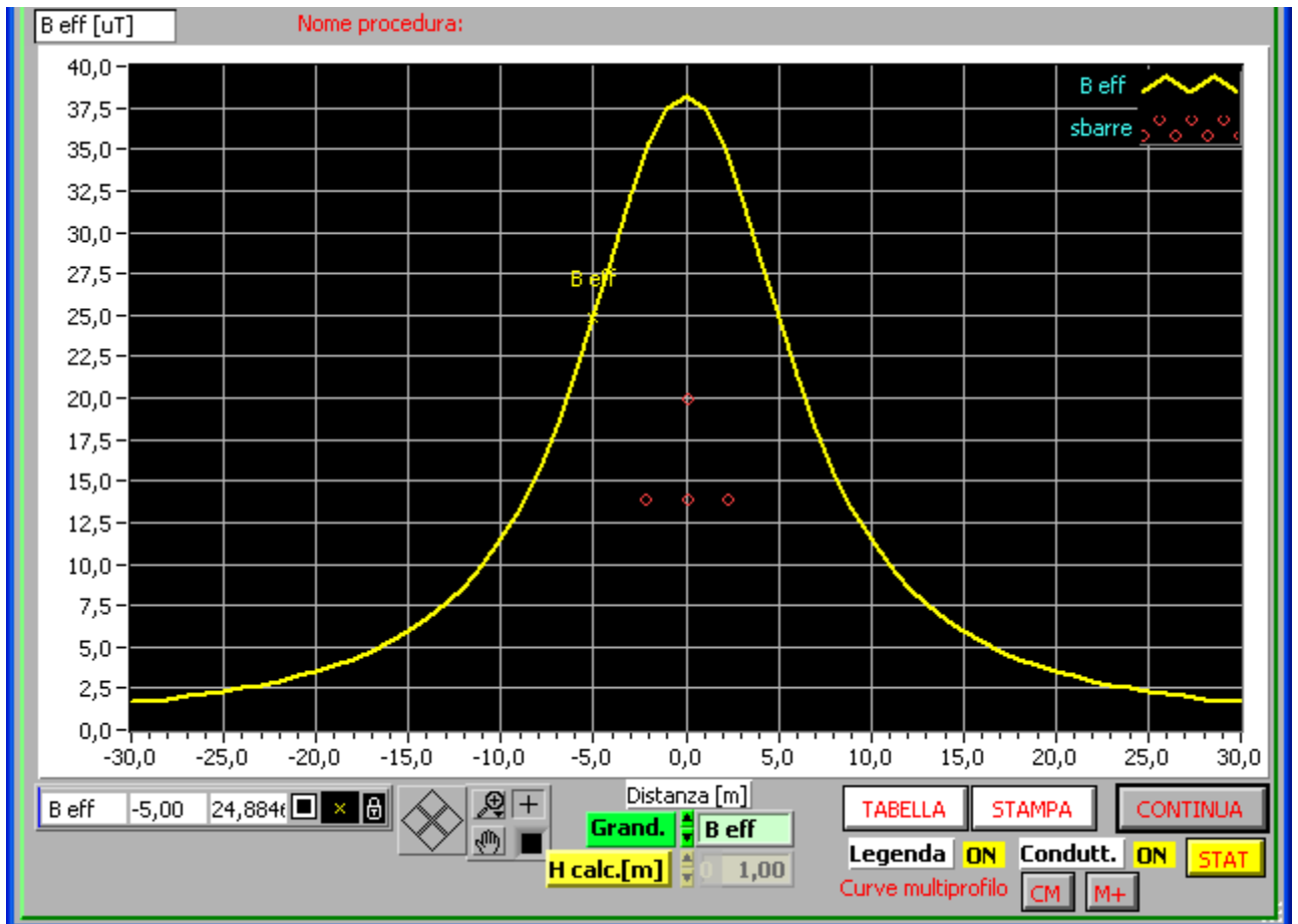
Figura 12: Andamento del campo di induzione magnetica per I = 2000\text{ A}
