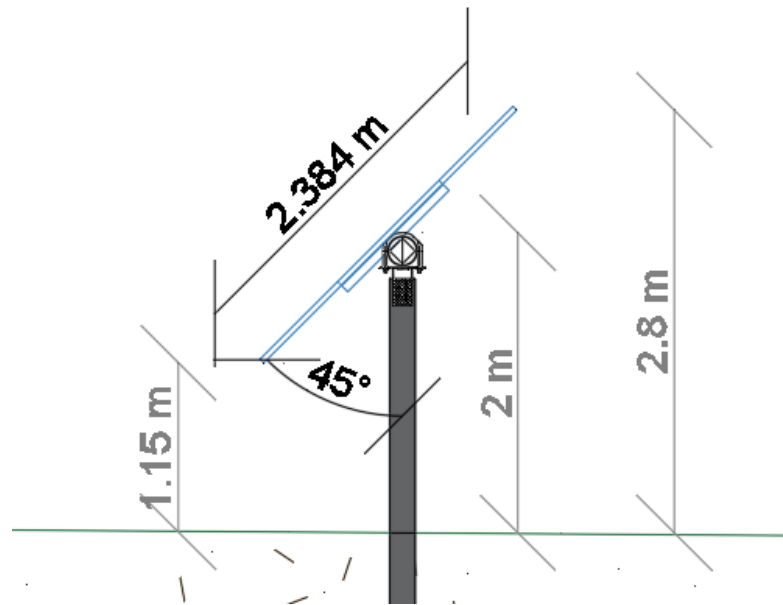
Struttura di supporto dei pannelli fotovoltaici
