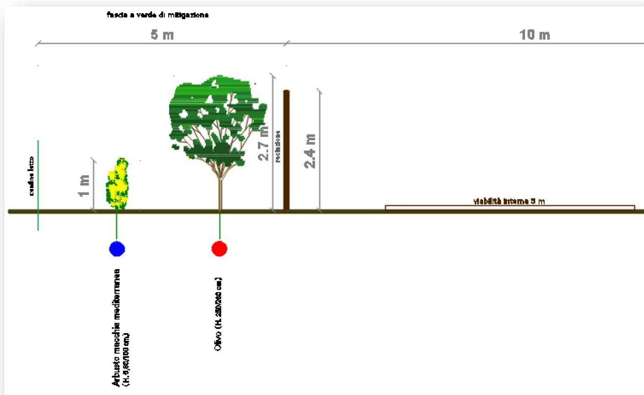
Stralcio sezione longitudinale opere mitigazione - tavola CV05
