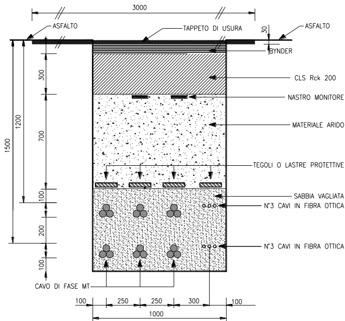
SEZIONE TIPO "HA"
