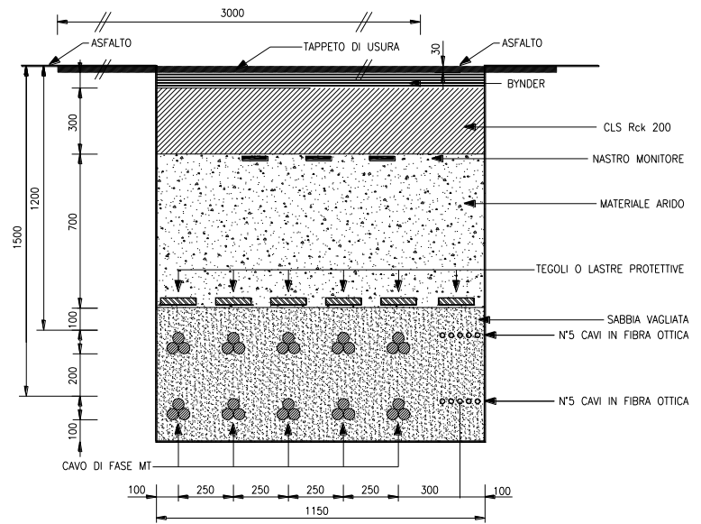
SEZIONE TIPO "JA"
