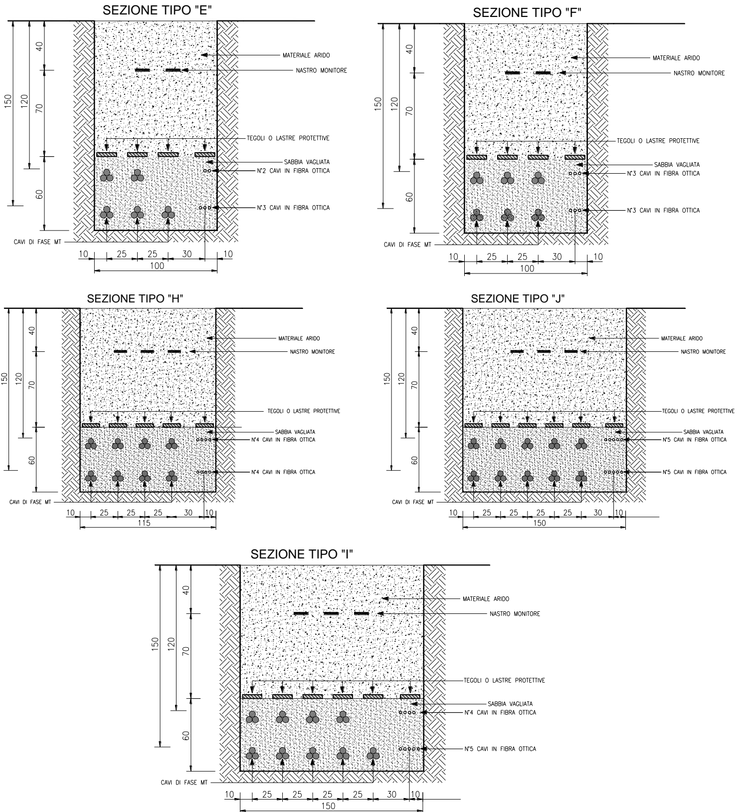
Figura 2: Sezione tipica di posa della linea in cavo su strada sterrata
