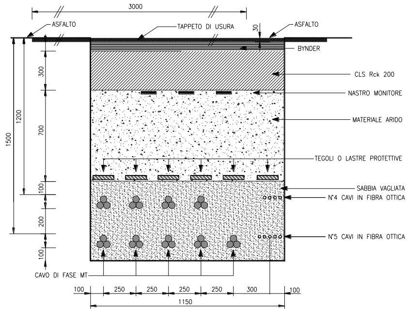
Figura 1: Sezione tipica di posa della linea in cavo su sede stradale
