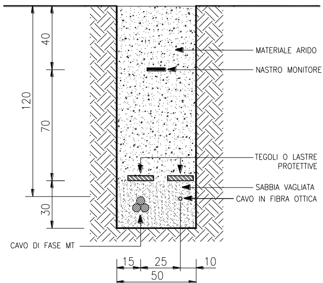
SEZIONE TIPO "A"
