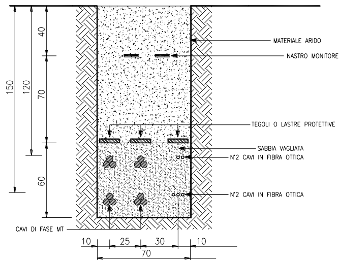
SEZIONE TIPO "D"
