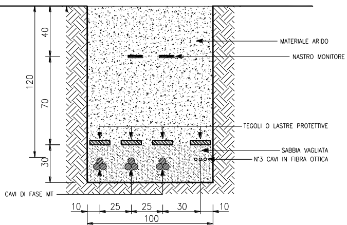
SEZIONE TIPO "C"
