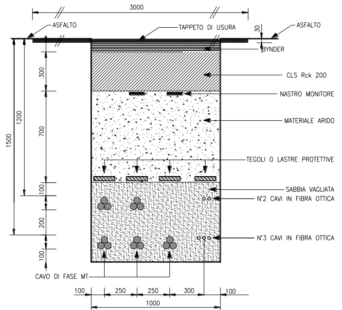
SEZIONE TIPO "JA"
