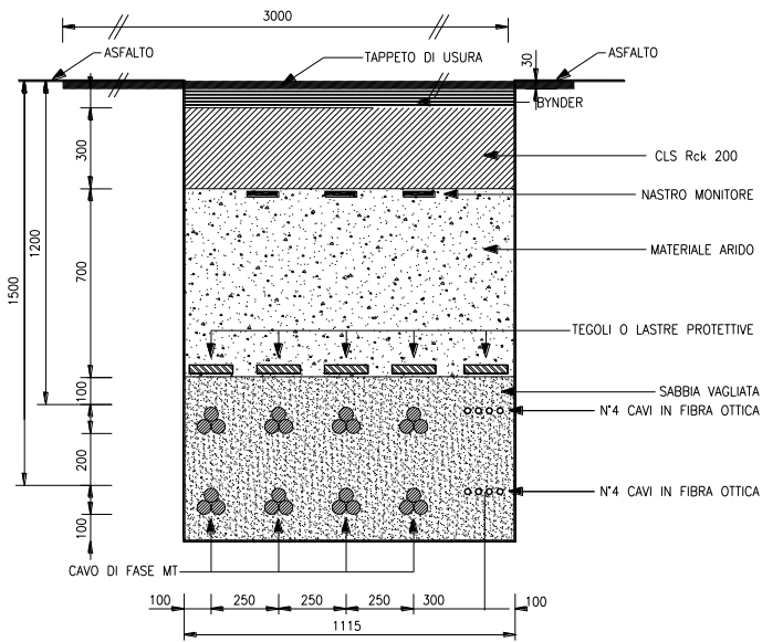
SEZIONE TIPO "HA"
