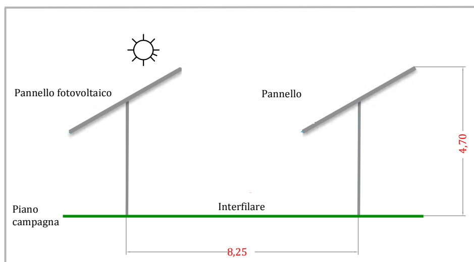
Sezione trasversale
