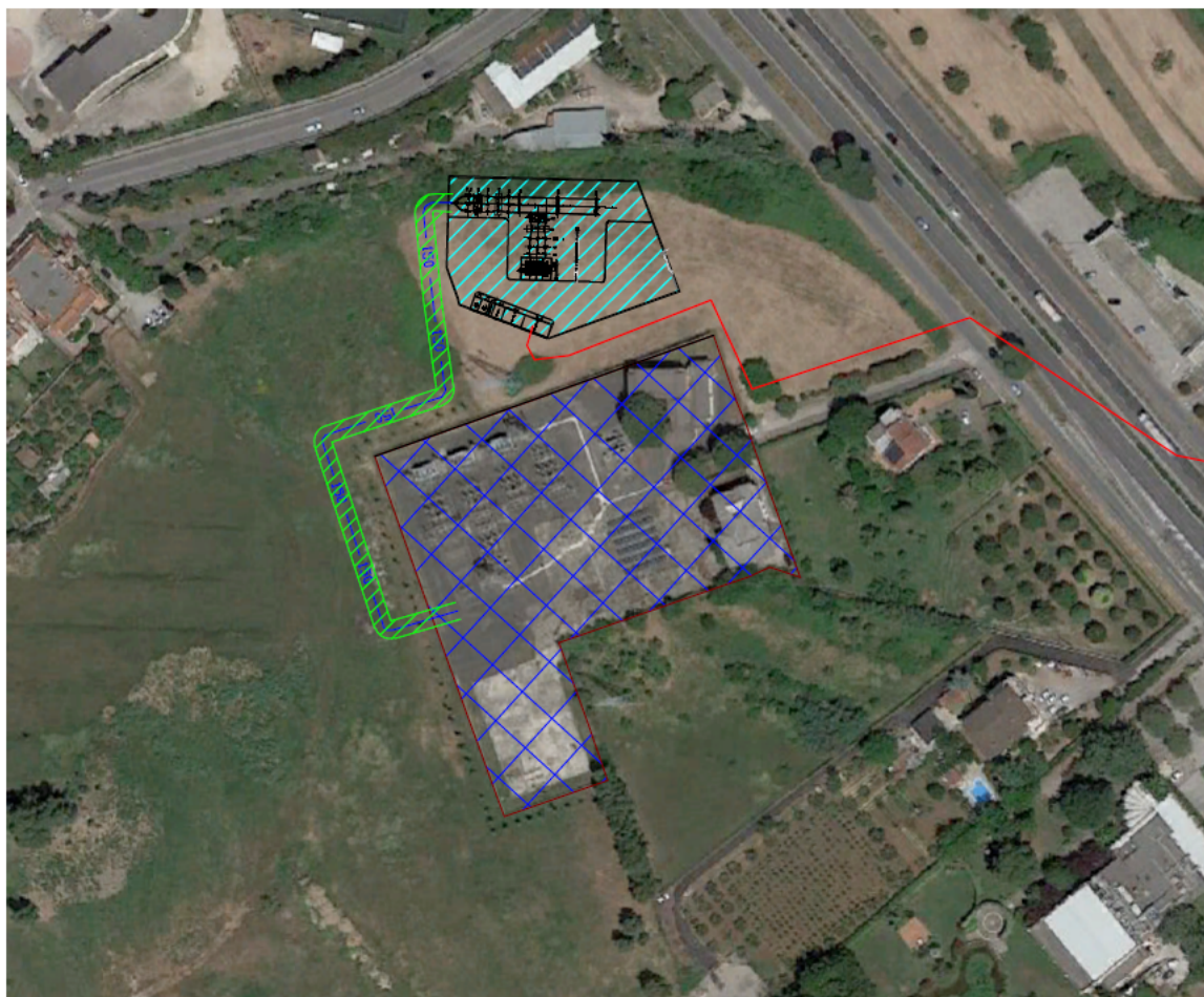
Tracciato cavidotto AT 150 kV su ortofoto
