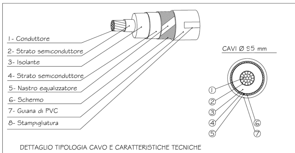
Componenti del cavo ARE4H1H5E 87/150 kV
