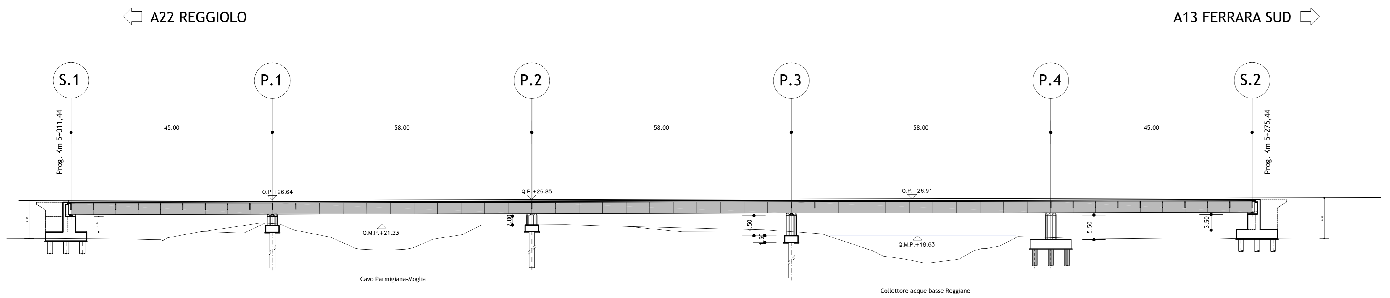
PROFILO LONGITUDINALE - 1:500
