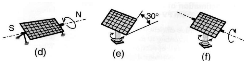
Movimenti degli Inseguitori Solari Monoassiali (b,c,d) e Biassiali (e,f)
