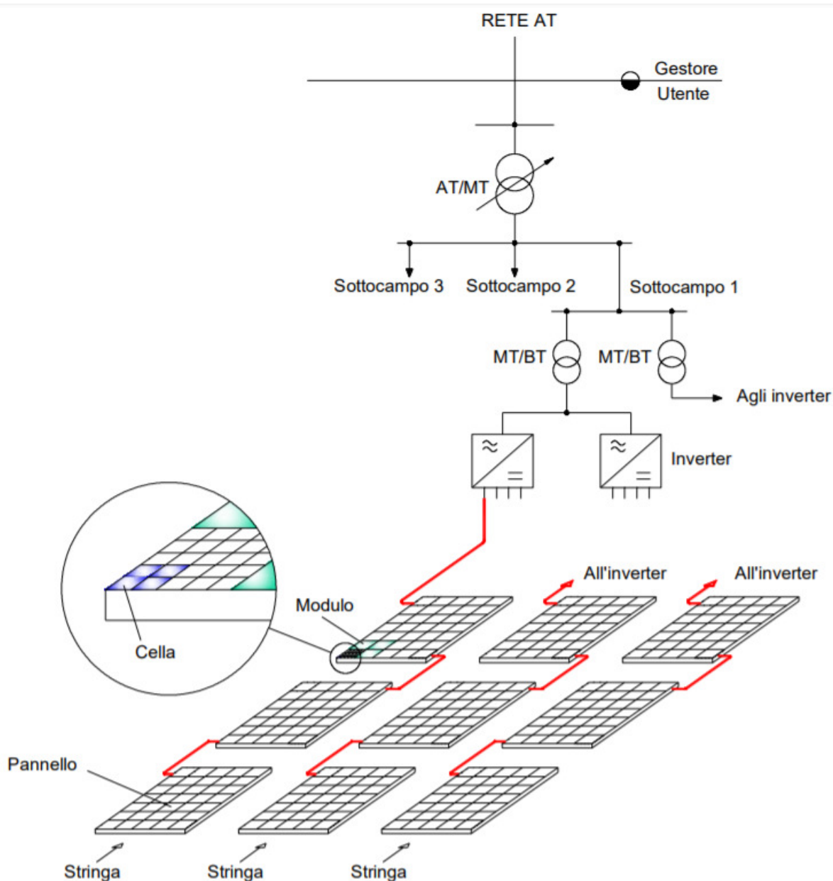
Schema sintetico della centrale di produzione solare di Trapani "Zaffarana 38")
