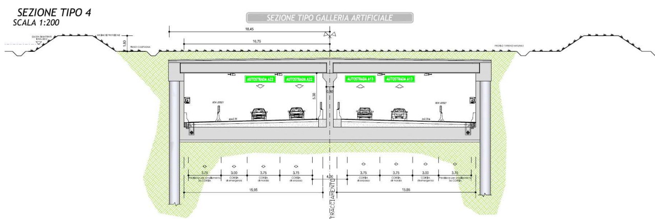
FIGURA 4.2-3 SEZIONE TIPO IN GALLERIA
