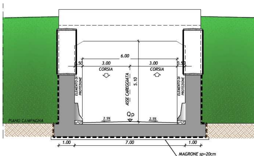
FIGURA 4.3-1 - SEZIONE TIPO SCATOLARE CHIUSO
