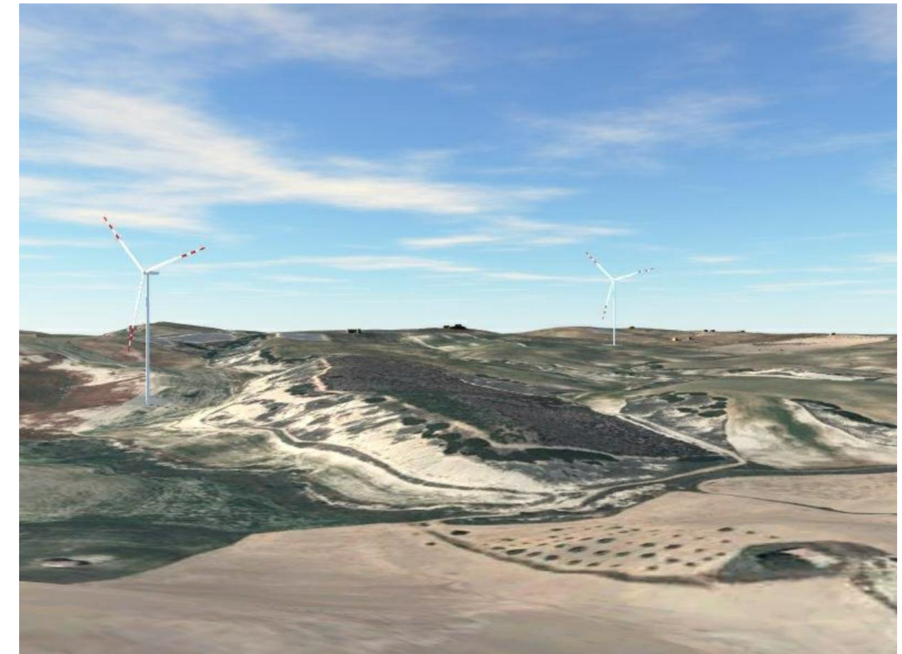
VISTA PANORAMICA AEROGENERATORI A4 - A5
