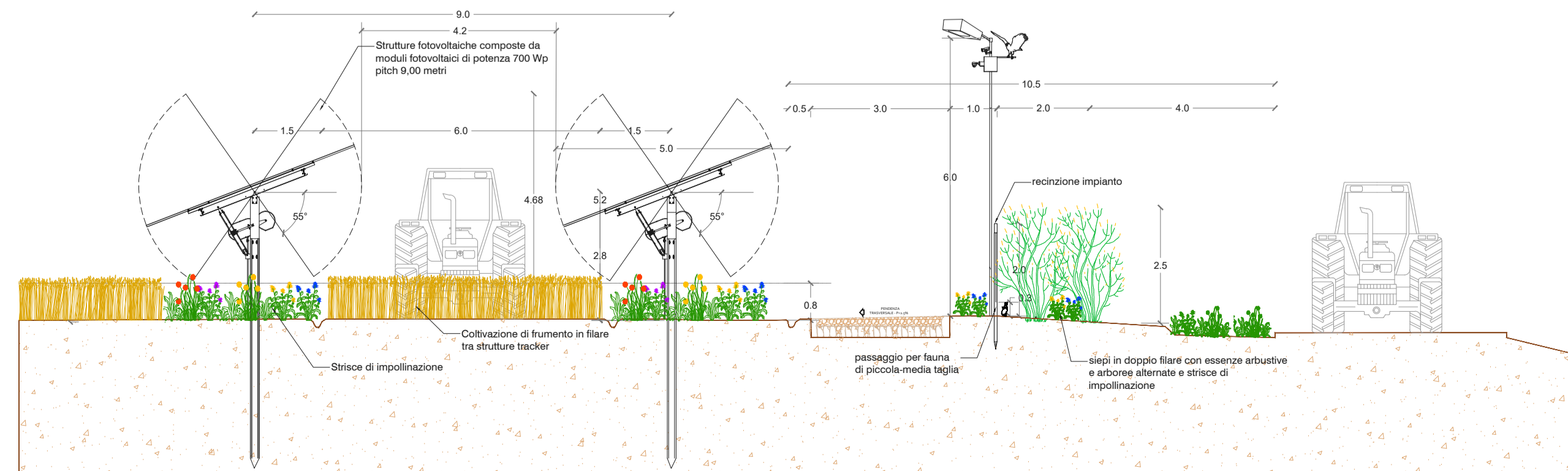
Sez. A - A'
