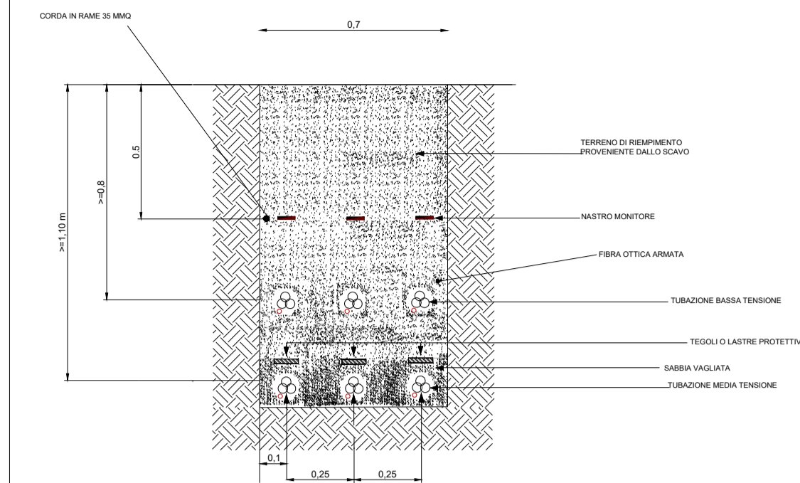
TIPICO SEZIONE DI SCAVO CAVI B.T. - M.T.: SCALA 1:20
