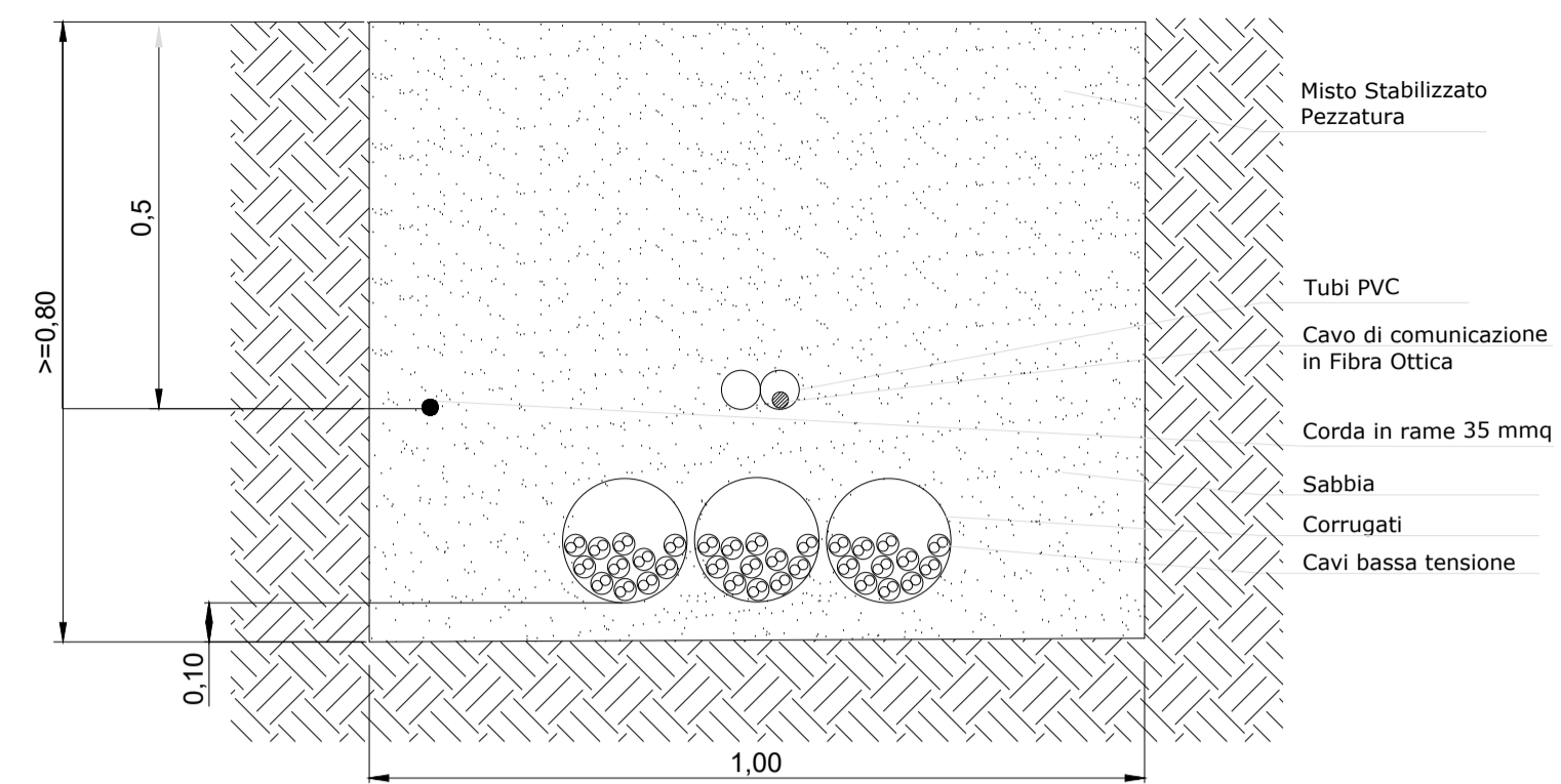
TIPICO SEZIONE DI SCAVO CAVI B.T.: SCALA 1:10
