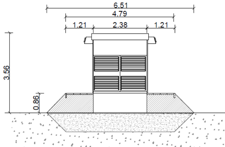
Figura 7: Prospetto laterale della cabina inverter
