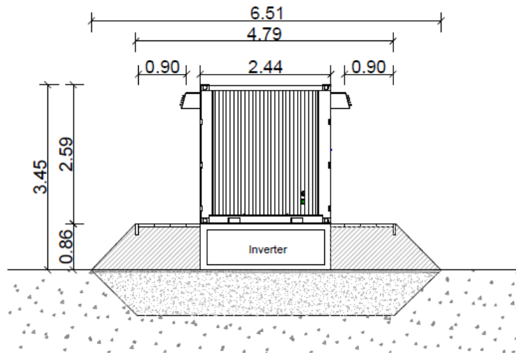
Figura 8: Prospetto laterale della cabina inverter
