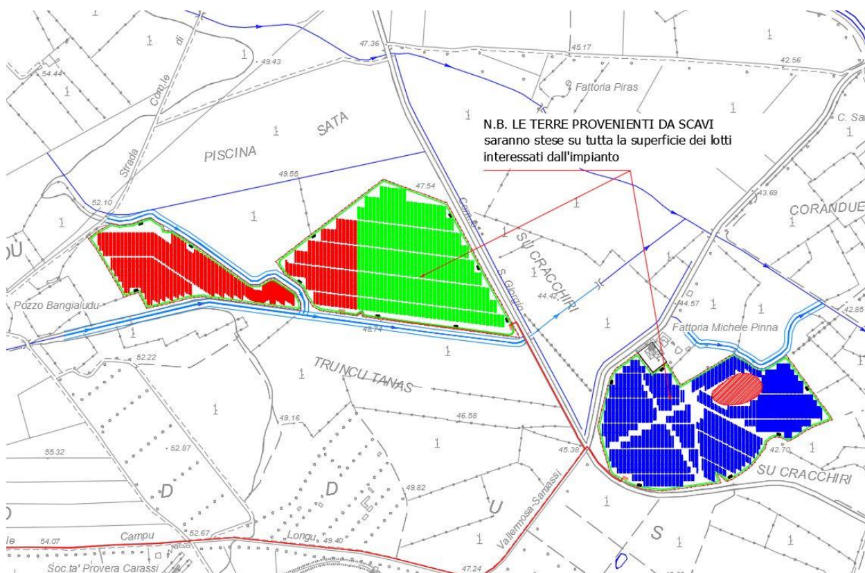
Fig. 1.1 Planimetria individuazione area spandimento terre da scavo
