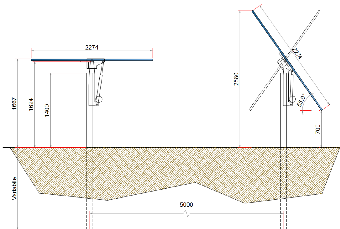
Fig. 2- Tracker - Inseguitore mono-assiale - intervalli di rotazione
