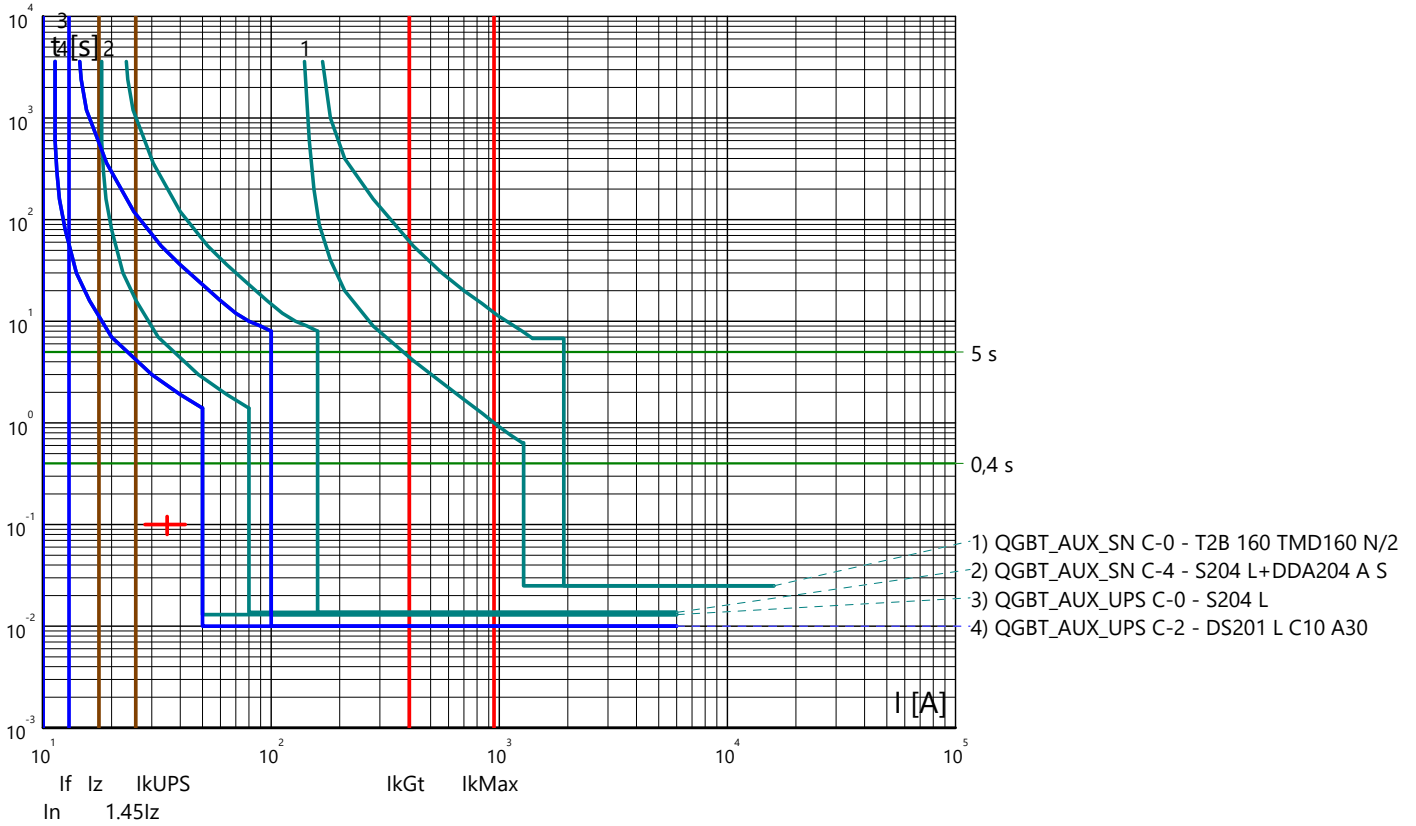
Partenza: QGBT_AUX_UPS C-2
