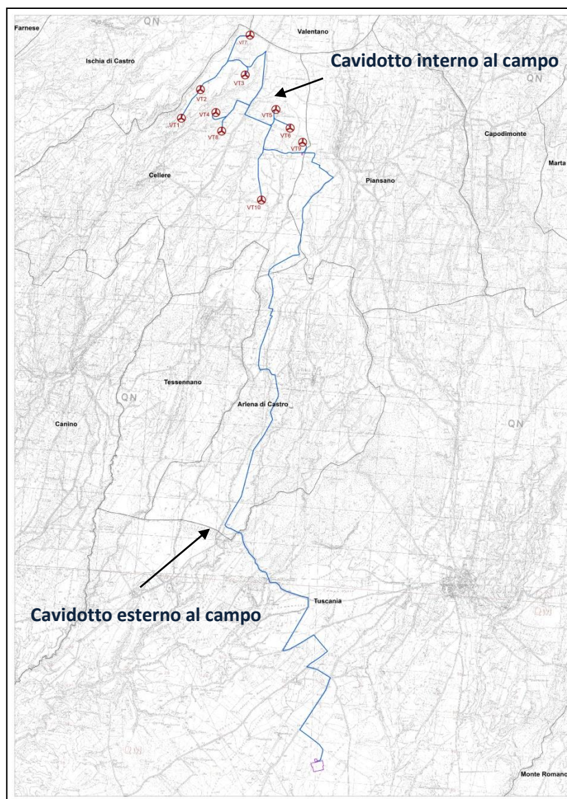
Figura 4 Rappresentazione del campo eolico e ubicazione delle opere connesse su CTR
