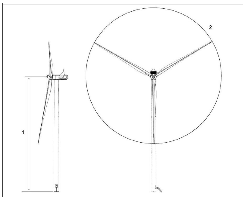
Figura 5 - Struttura Vestas V162
