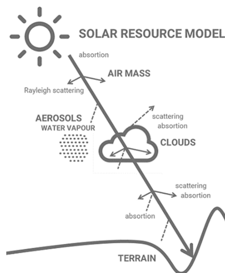
Figura 3.1 – Parametri del modello di radiazione solare Solargis.
