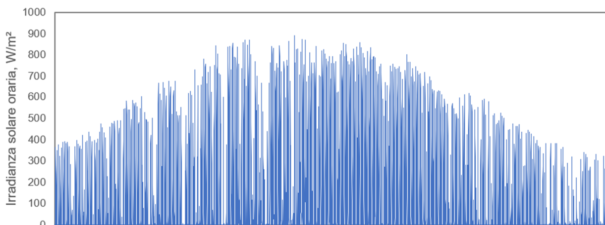
Figura 3.5 – Serie storica oraria dell'irradianza solare globale su superficie orizzontale.
