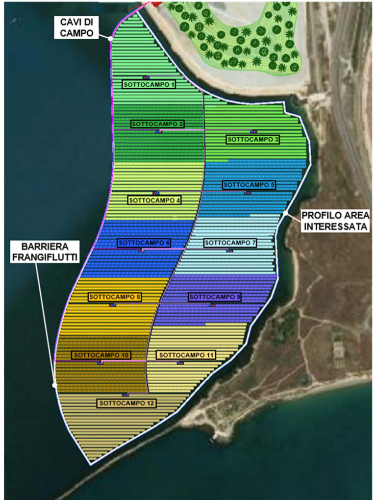
Figura 4.1 – Layout di impianto impiegato per le analisi di producibilità energetica. Elaborazione iLStudio.
