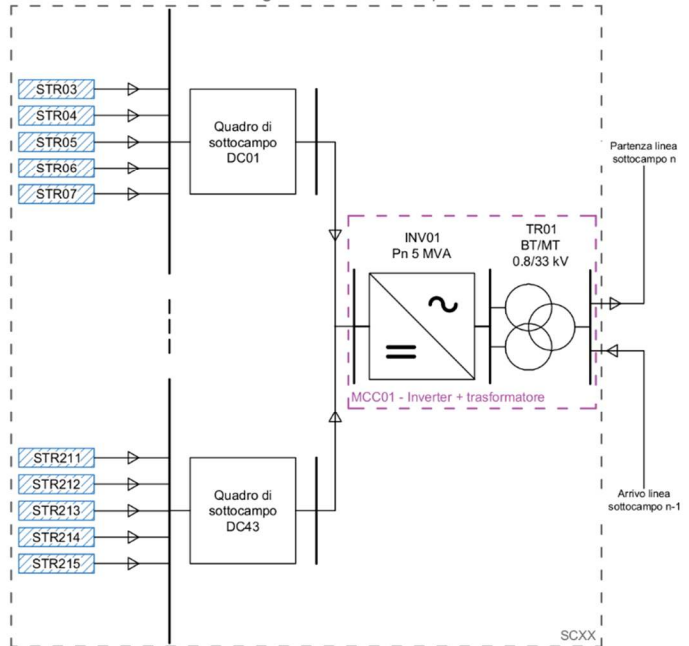
Figura 5.3 – Schema a blocchi dell'architettura elettrica del parco fotovoltaico.
