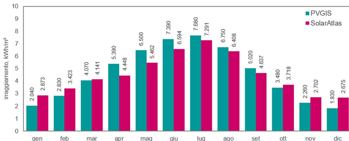
Figura 3.6 – Irraggiamento gionaliero medio mensile su superficie normale ai raggi. Confronto tra i dataset Global Solar Atlas e PVGIS.
