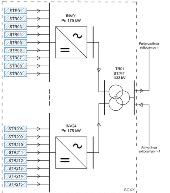
Figura 5.3 – Schema a blocchi dell'architettura elettrica del parco fotovoltaico.
