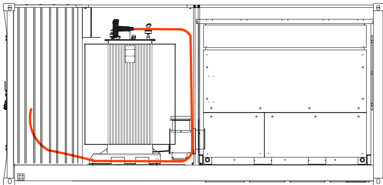
PROSPETTO "B"
