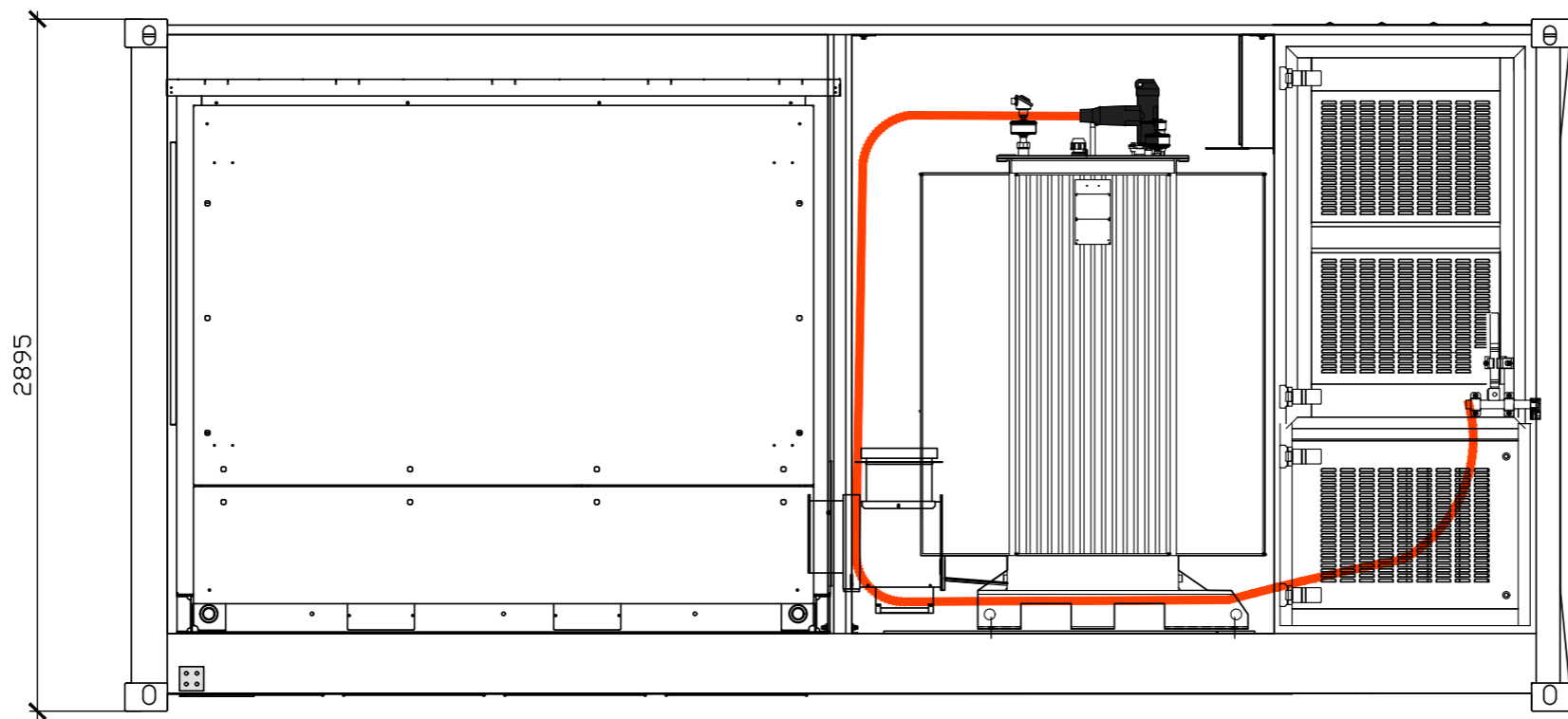
PROSPETTO "A"
