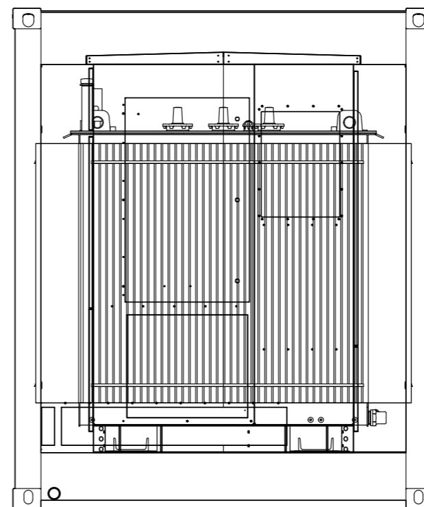
PROSPETTO "D"
