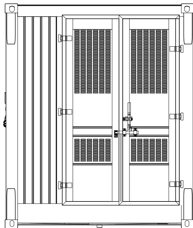
PROSPETTO "B"
