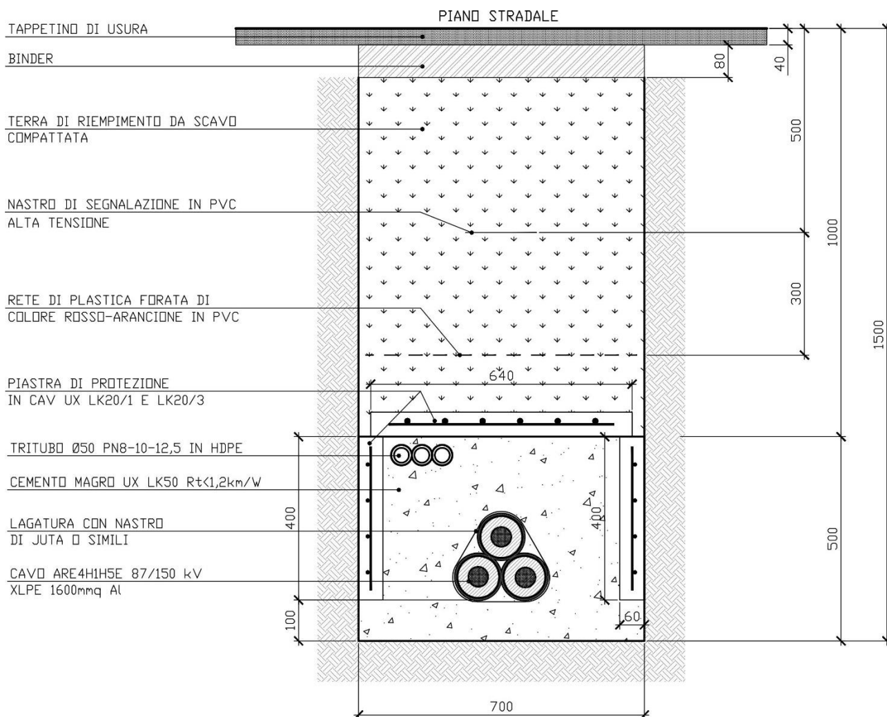
Figura 4 - Sezione di posa a trifoglio sotto strada
