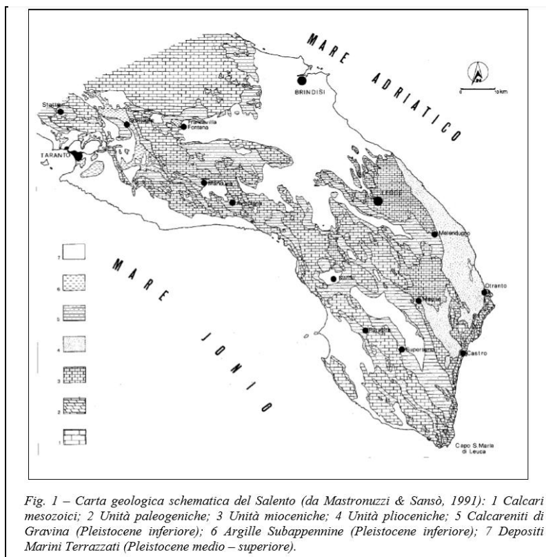
Figura 5 Carta geologica schematica del Salento (MASTRONUZZI- SANSO' 1991)
