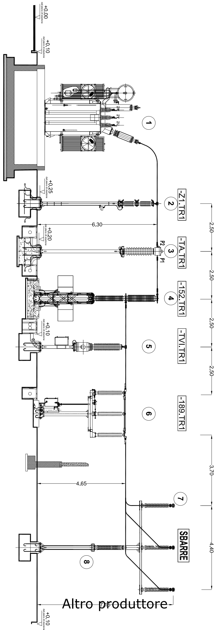
SEZ.A
