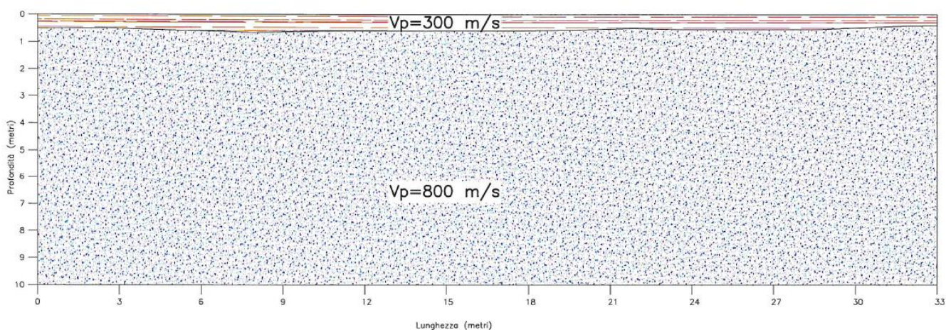
PROFILO SISMICO A RIFRAZIONE 1-1' LOCALITÀ: CERIGNOLA (FG)
