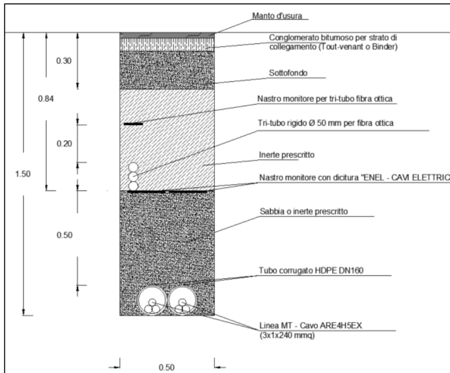
Figura 3 - Tipologico di posa dei cavidotti due terne di cavi nello stesso scavo
