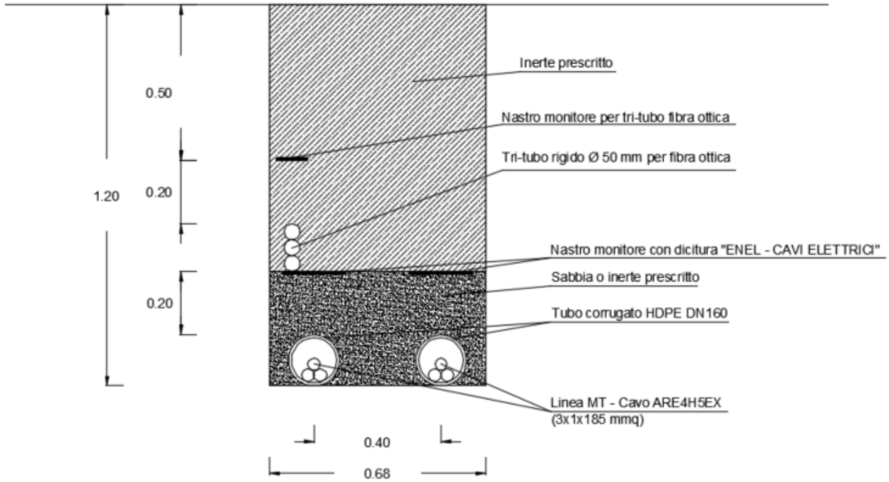
Figura 3 – Tipologico di posa dei cavidotti due terne di cavi nello stesso scavo
