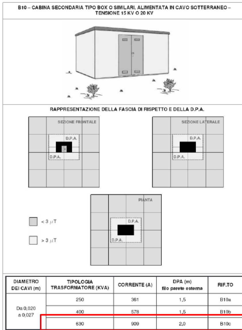
Figura 4 – Stralcio della "Linea Guida per l'applicazione del § 5.1.3 dell'Allegato al DM 29.05.08" di e-Distribuzione con indicazione della DPA prevista per cabine di tipo box alimentate da cavi sotterranei
